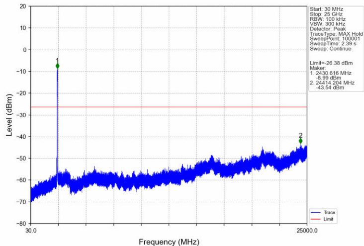
802.11n(HT40)_MCH_2437MHz_Ant1 (SISO)_NTNV
