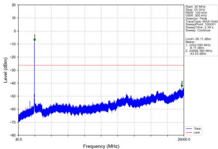
802.11n(HT40)_MCH_2437MHz_Ant1 (SISO)_NTNV
