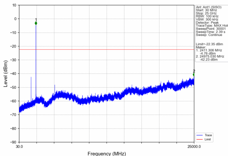
802.11b_LCH_2412MHz_Ant1 (SISO)_NTNV
