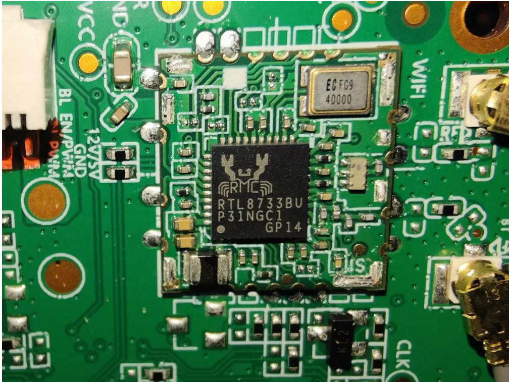
Internal Photos(K200)
