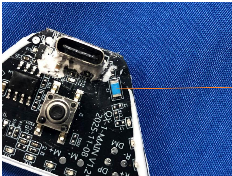
BLE ANT
