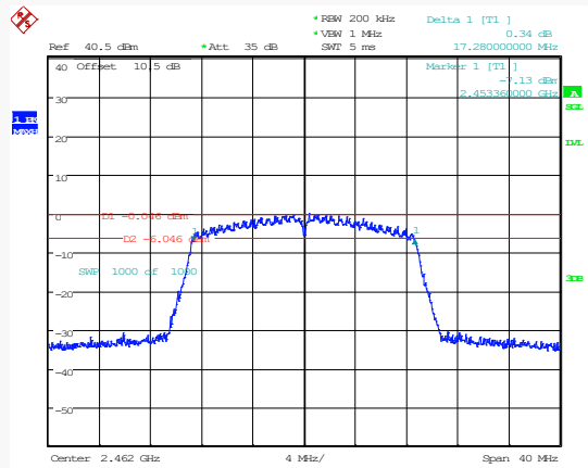
802.11n20_2462MHz
