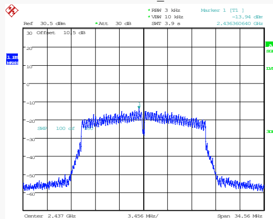
802.11n20_2437MHz
