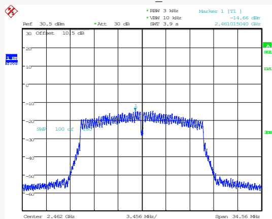
802.11n20_2462MHz
