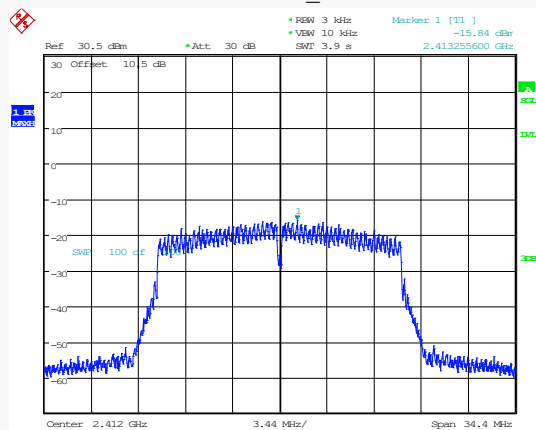
802.11n20_2412MHz
