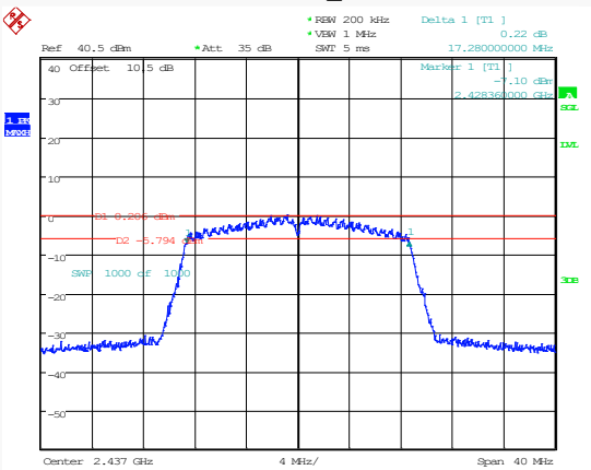
802.11n20_2437MHz
