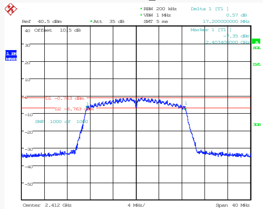
802.11n20_2412MHz
