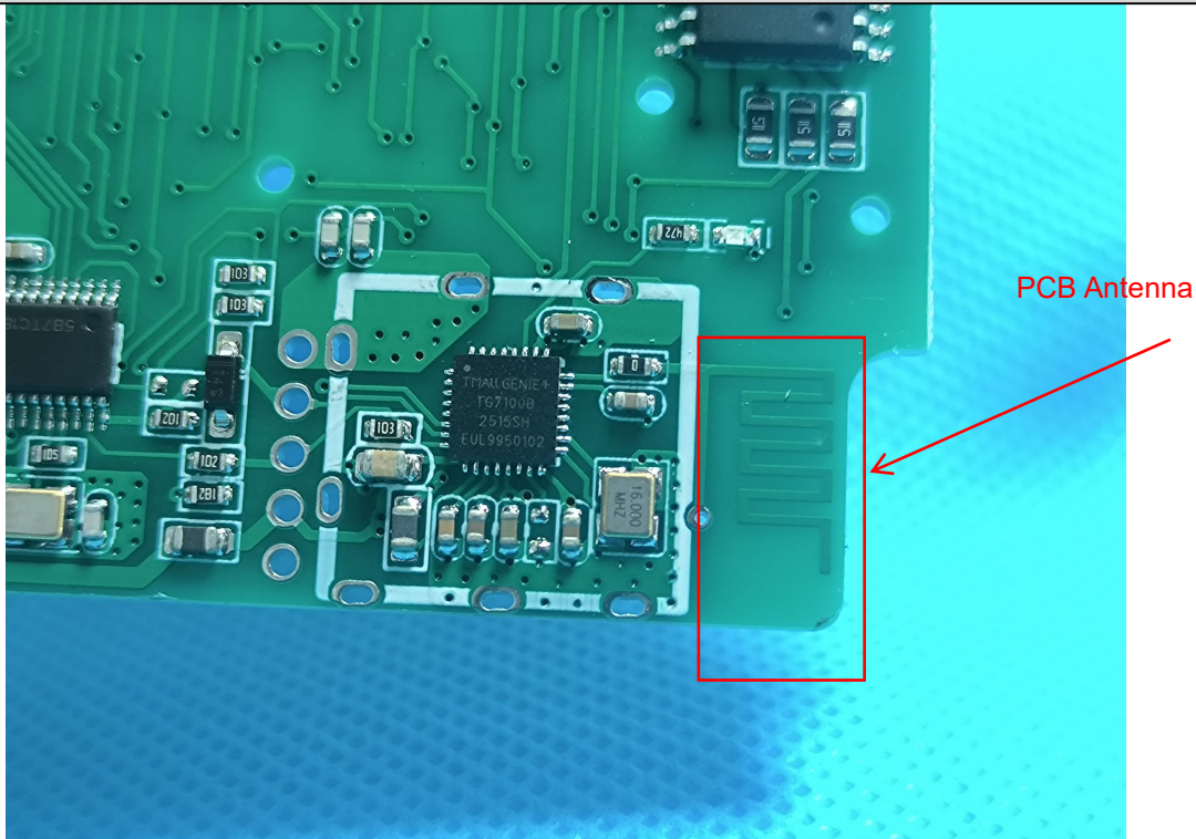
EUT Photo
