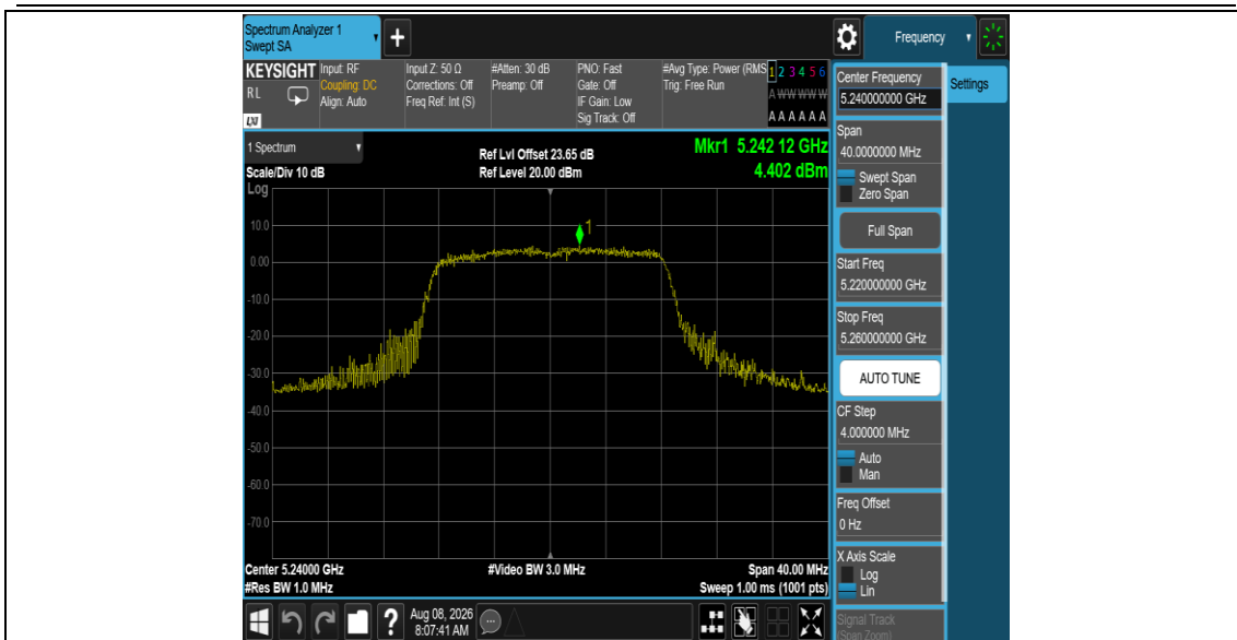
11A_Ant1_5240
