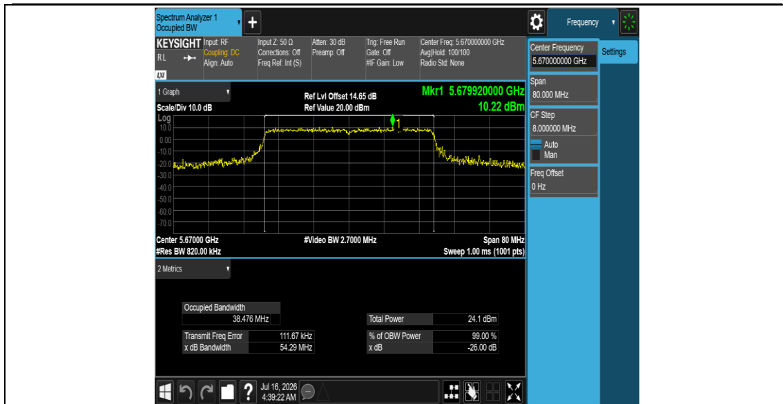
11AX40SISO_Ant1_5670
