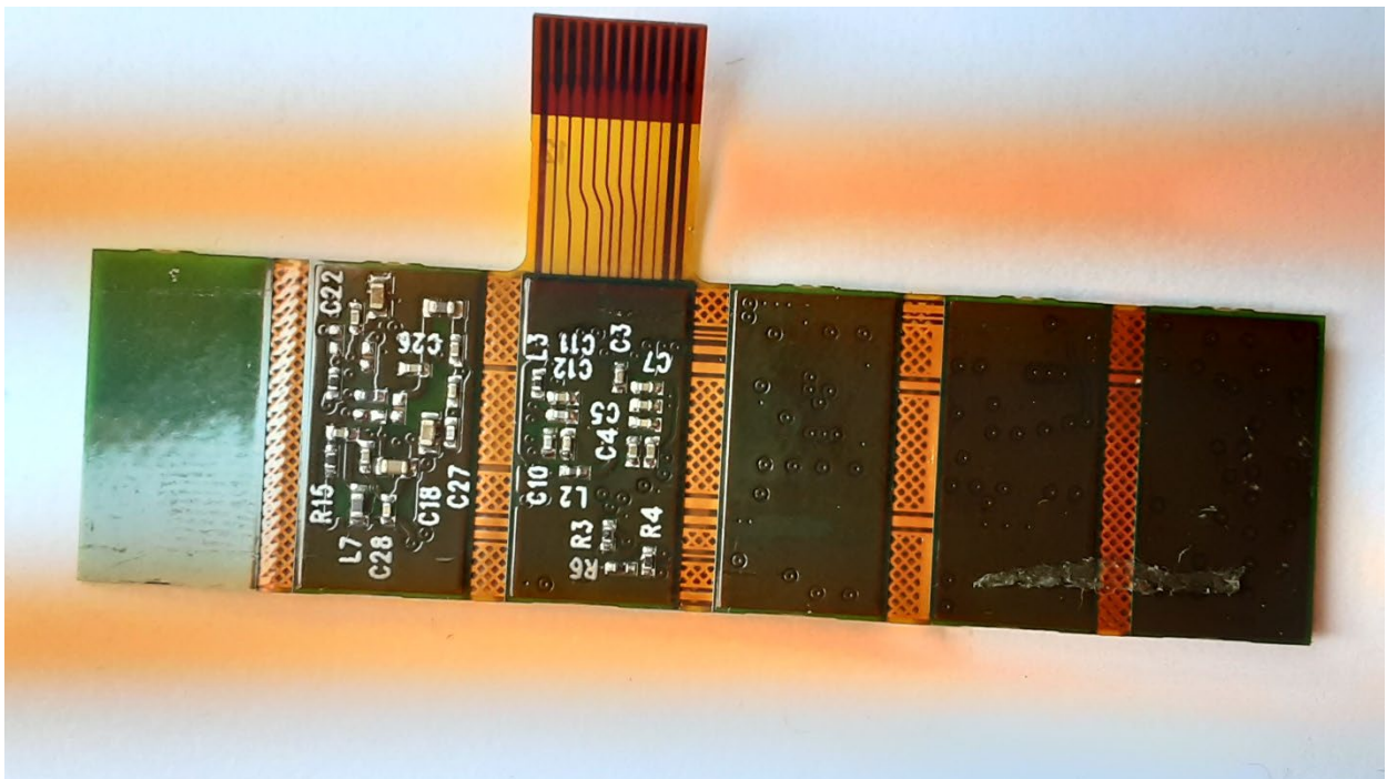
PCB Bottom
