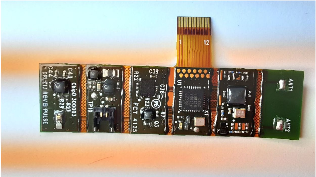
PCB Top
