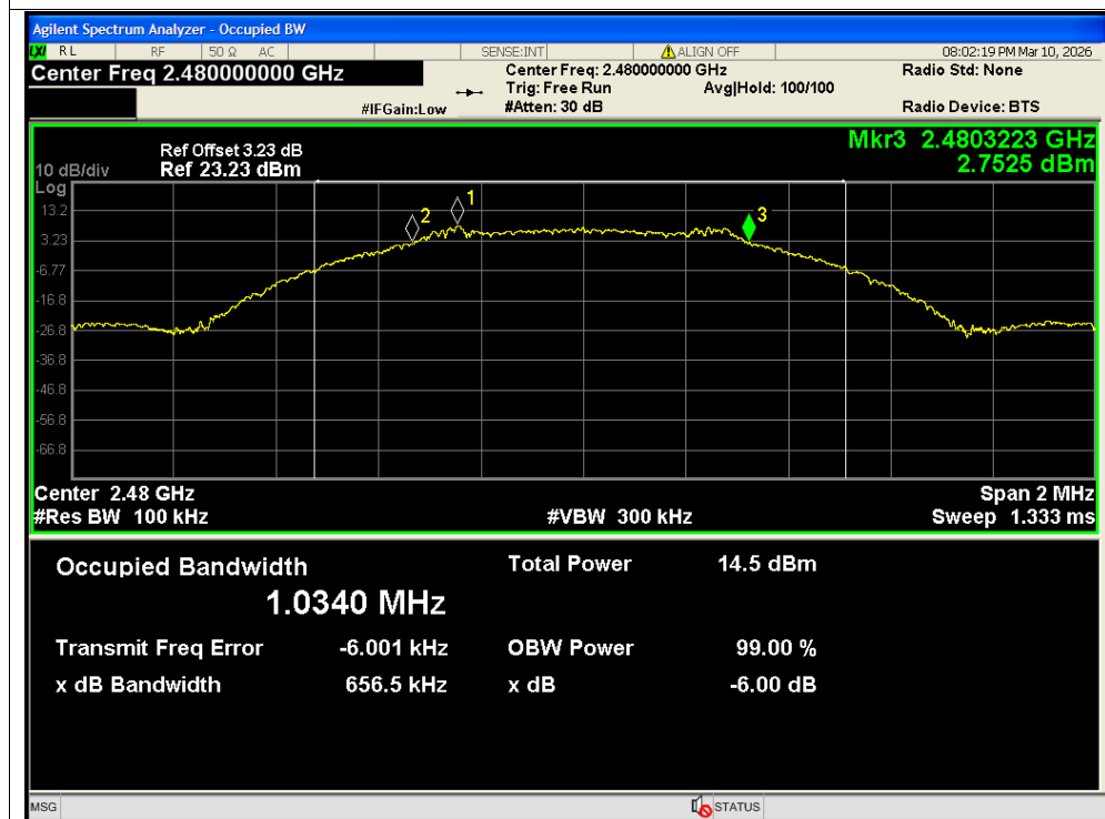
-6dB Bandwidth NVNT BLE 1M 2480MHz Ant2
