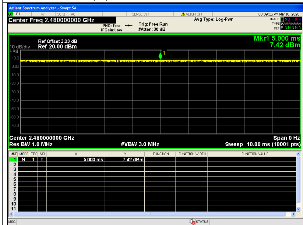
Duty Cycle NVNT BLE 2M 2480MHz Ant2
