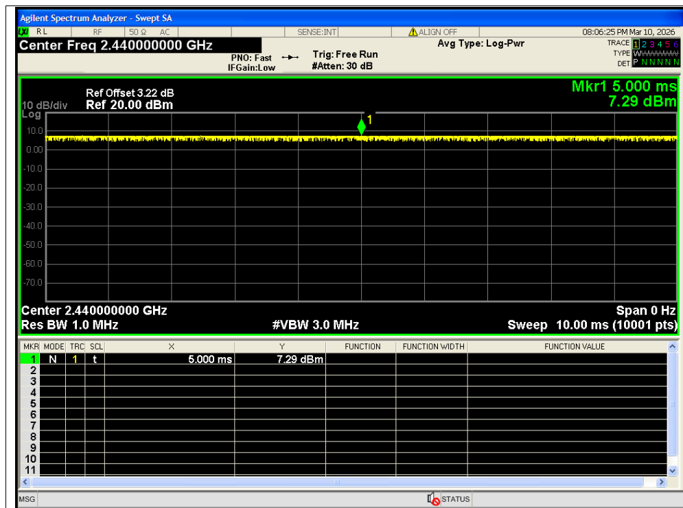
Duty Cycle NVNT BLE 2M 2440MHz Ant2
