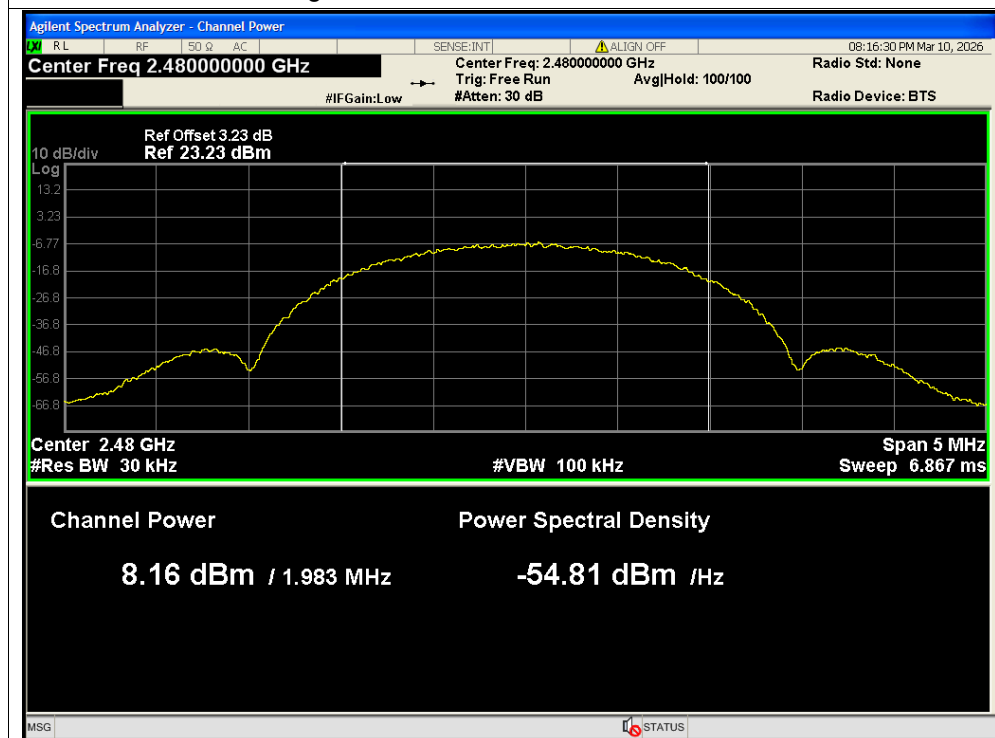
Average Power NVNT BLE 2M 2480MHz Ant2
