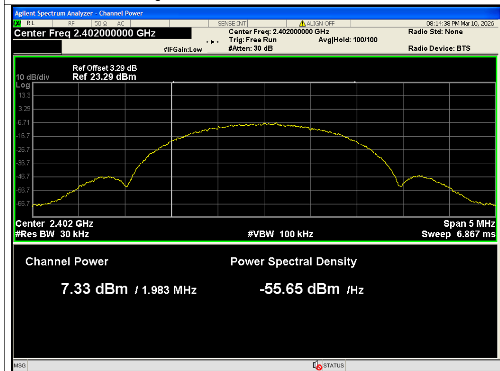
Average Power NVNT BLE 2M 2402MHz Ant2
