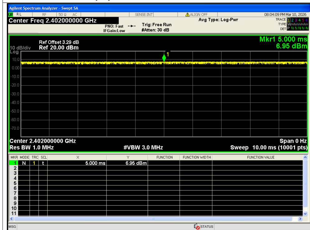
Duty Cycle NVNT BLE 2M 2402MHz Ant2
