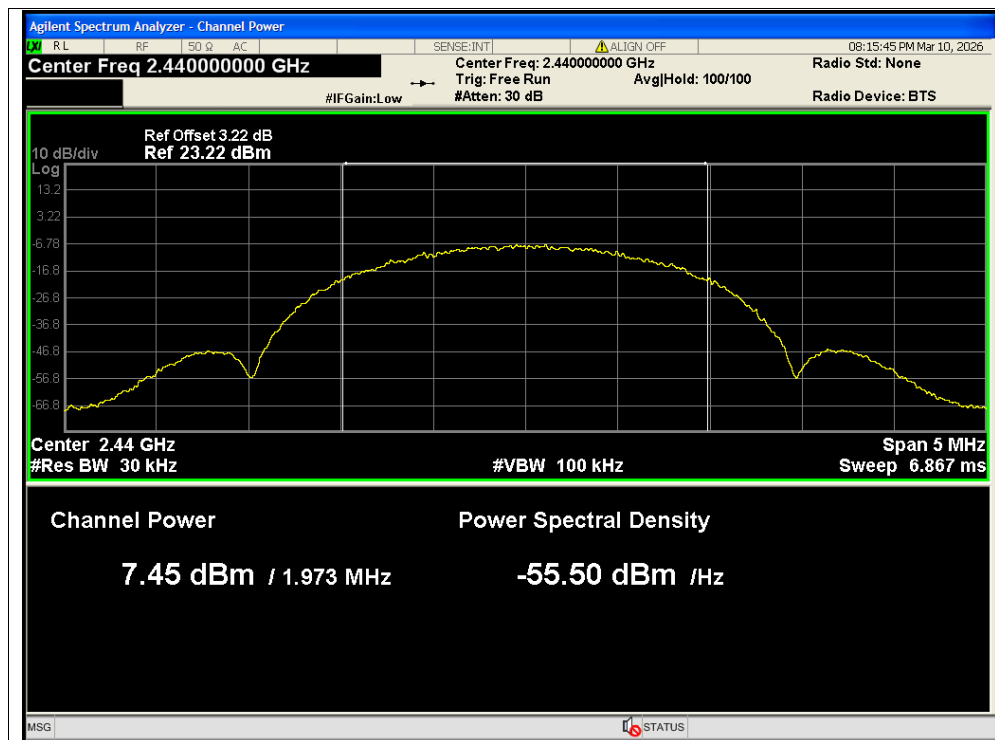
Average Power NVNT BLE 2M 2440MHz Ant2
