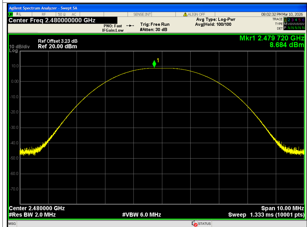
Peak Power NVNT BLE 1M 2480MHz Ant2
