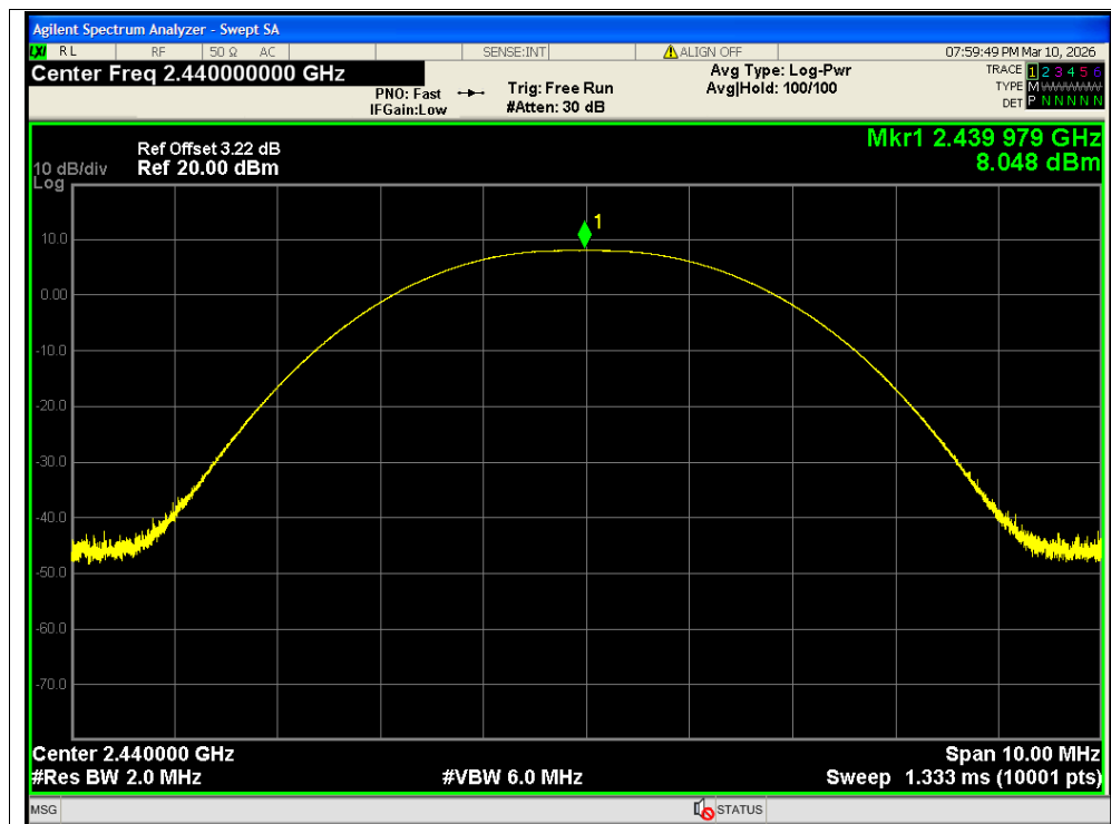
Peak Power NVNT BLE 1M 2440MHz Ant2
