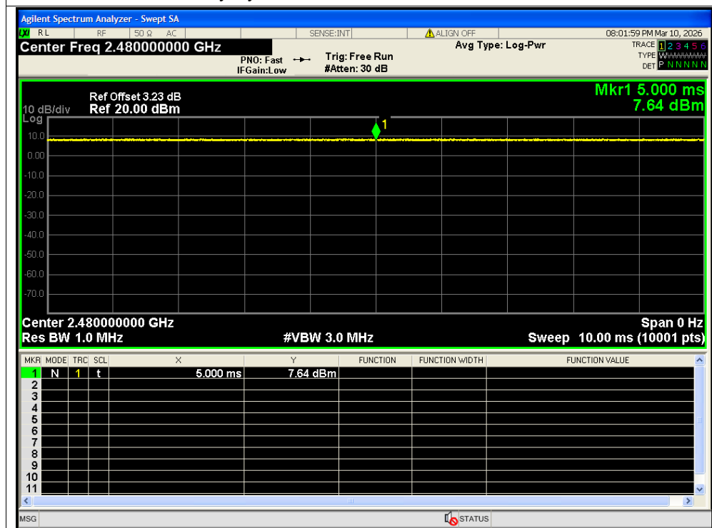
Duty Cycle NVNT BLE 1M 2480MHz Ant2
