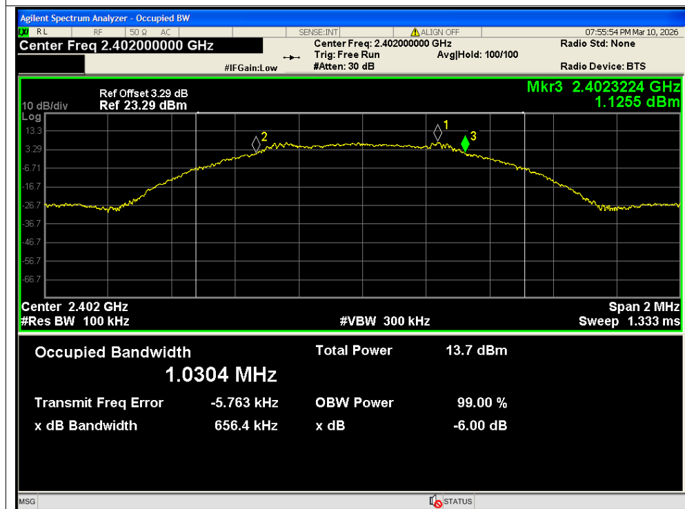
-6dB Bandwidth NVNT BLE 1M 2402MHz Ant2
