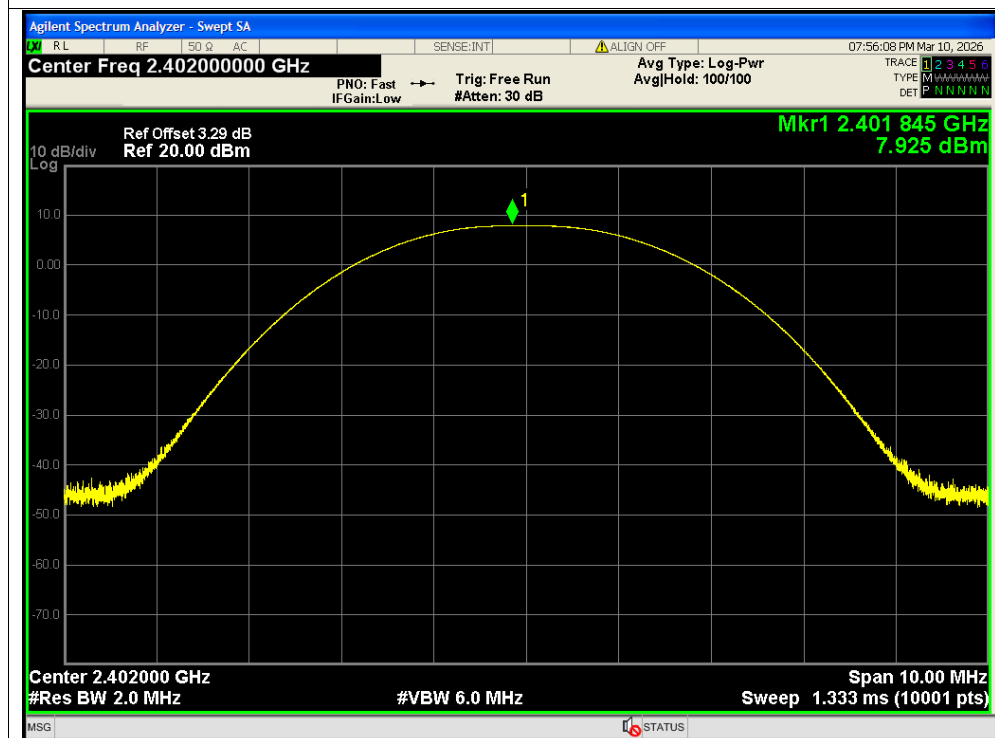
Peak Power NVNT BLE 1M 2402MHz Ant2
