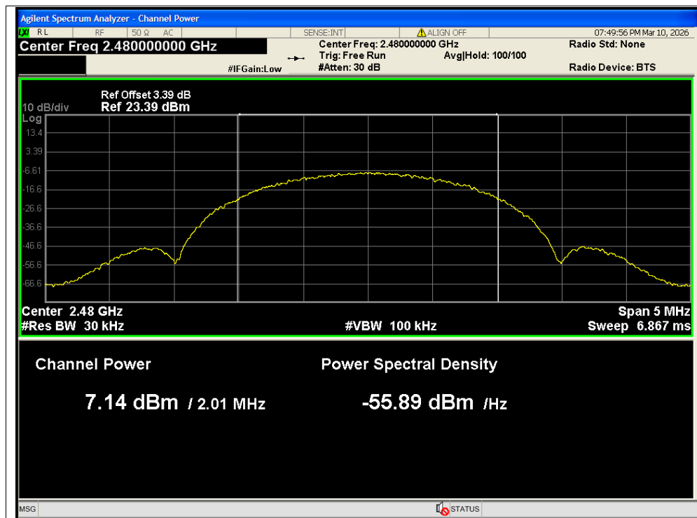
Average Power NVNT BLE 2M 2480MHz Ant1
