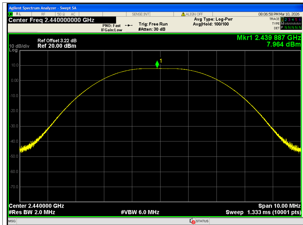
Peak Power NVNT BLE 2M 2440MHz Ant2
