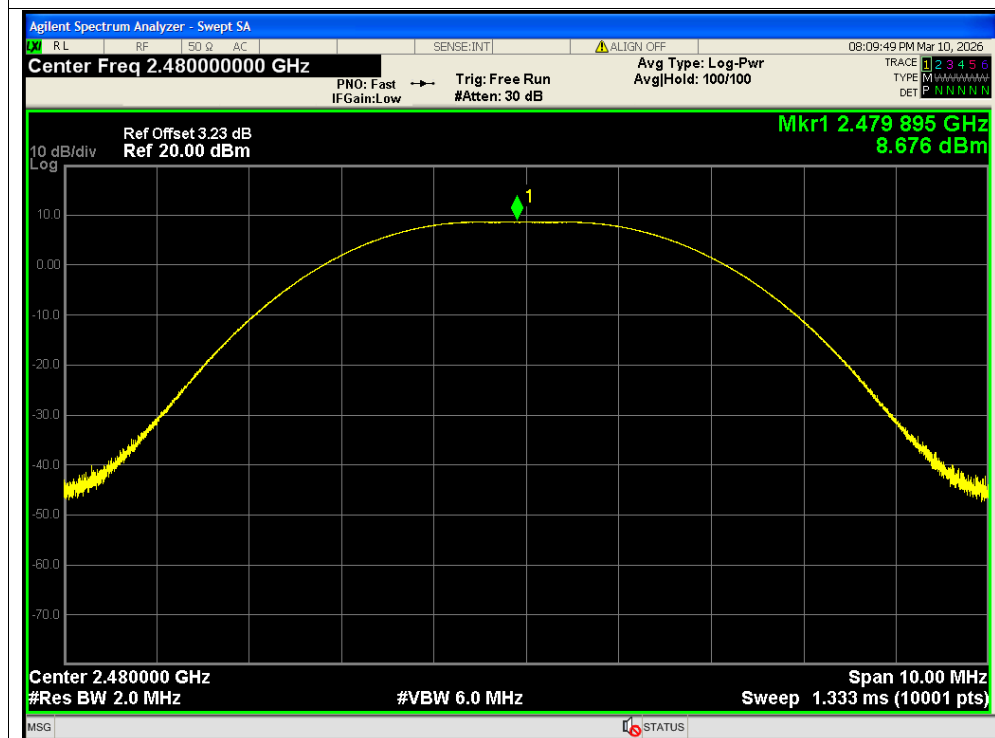
Peak Power NVNT BLE 2M 2480MHz Ant2
