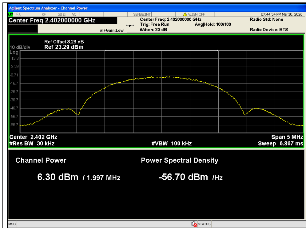
Average Power NVNT BLE 2M 2402MHz Ant1
