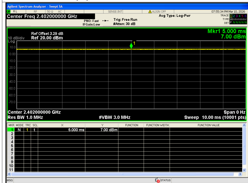
Duty Cycle NVNT BLE 1M 2402MHz Ant2
