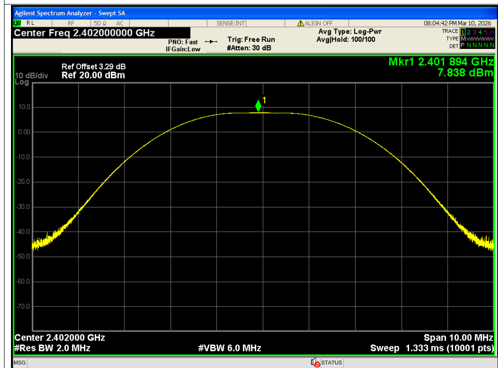
Peak Power NVNT BLE 2M 2402MHz Ant2
