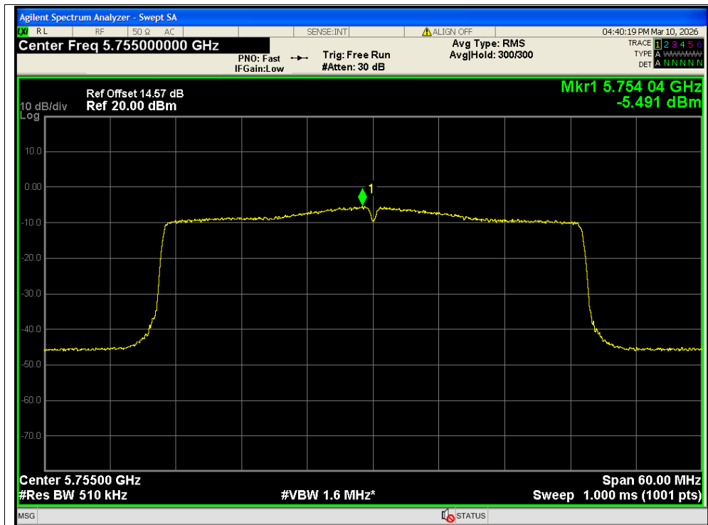
PSD NVNT ax40 5755MHz Ant1 MIMO
