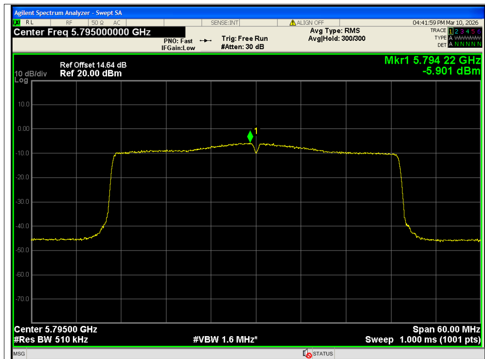
PSD NVNT ax40 5795MHz Ant1 MIMO
