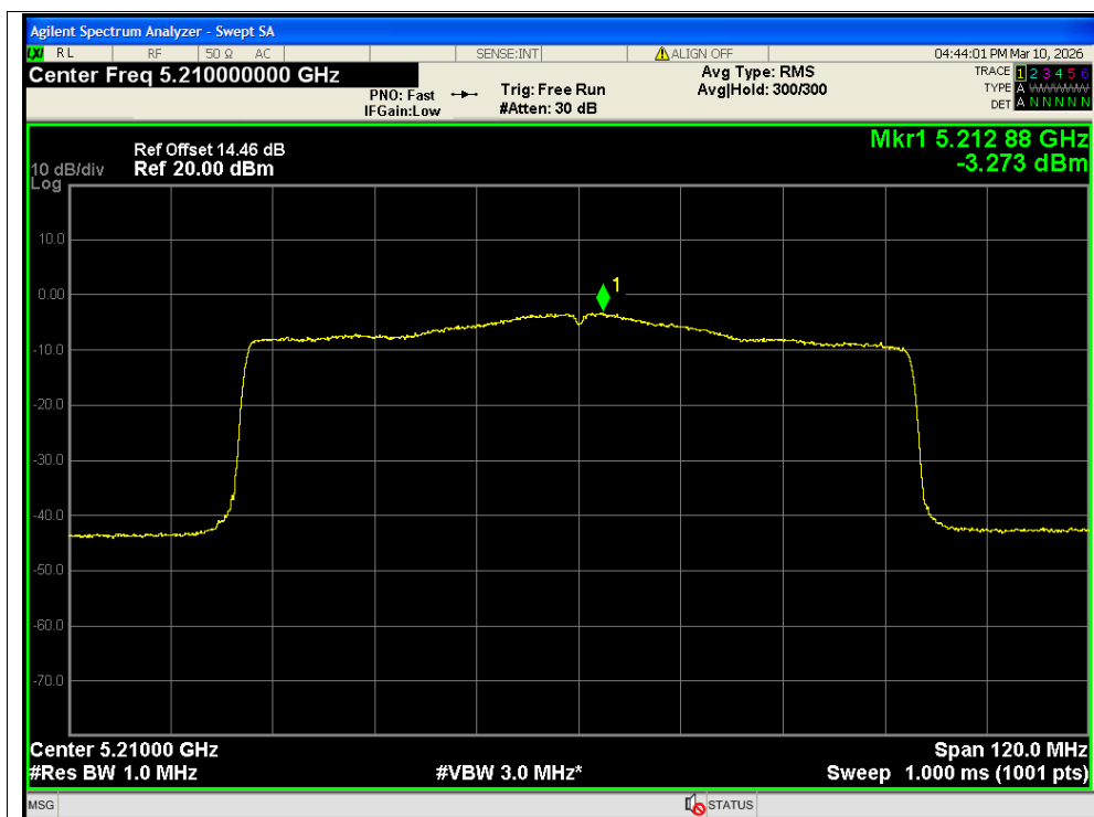
PSD NVNT ax80 5210MHz Ant1 MIMO
