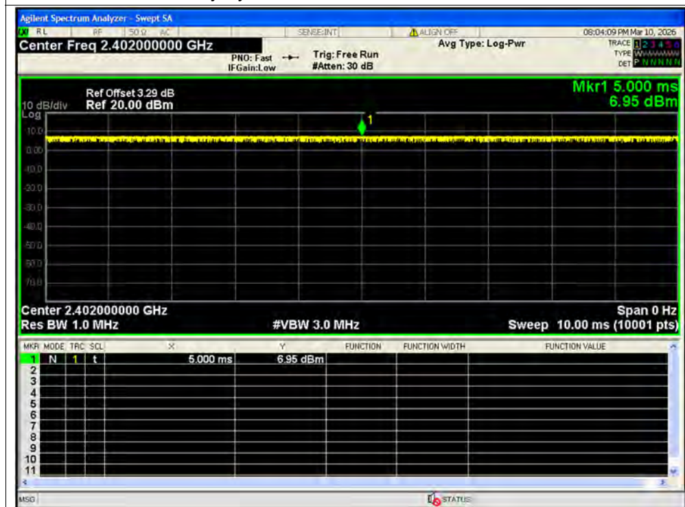
Duty Cycle NVNT BLE 2M 2402MHz Ant2
