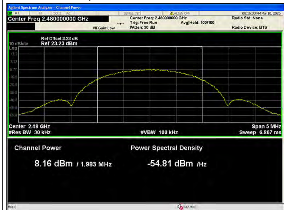
Average Power NVNT BLE 2M 2480MHz Ant2
