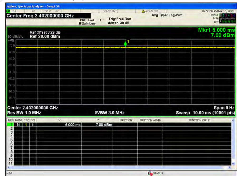
Duty Cycle NVNT BLE 1M 2402MHz Ant2
