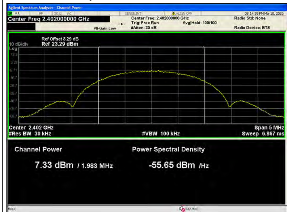
Average Power NVNT BLE 2M 2402MHz Ant2
