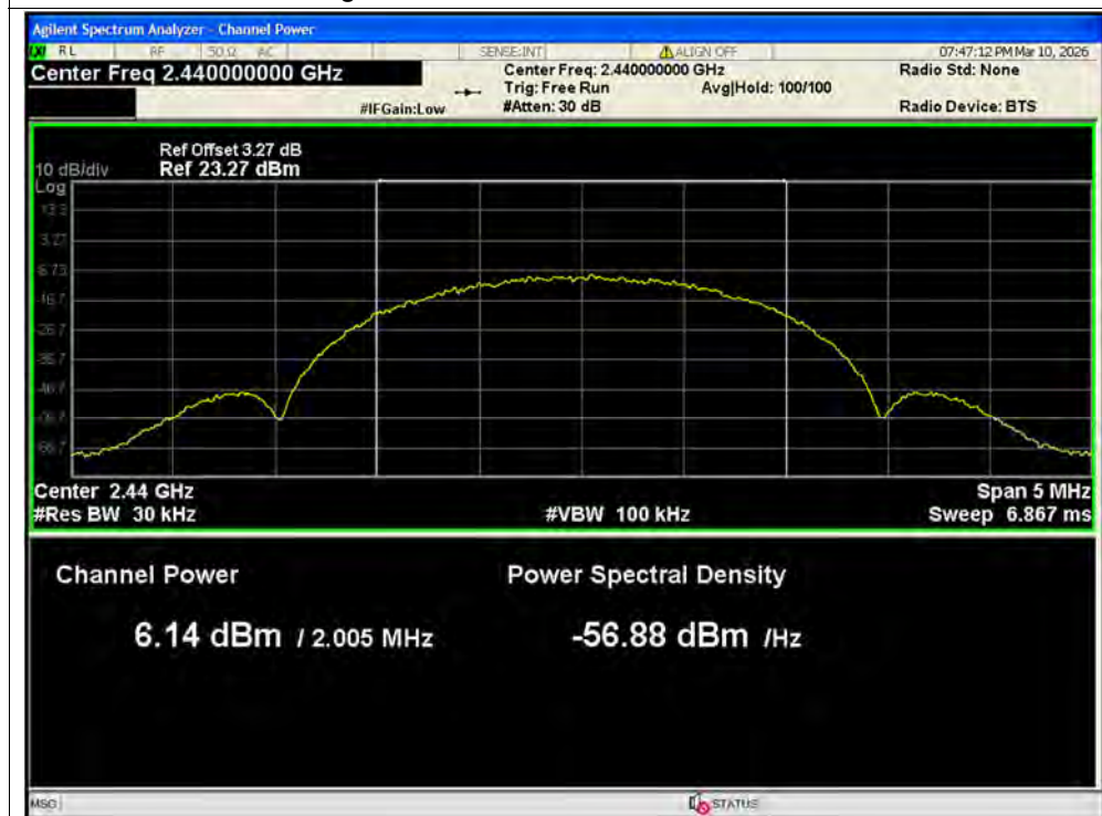
Average Power NVNT BLE 2M 2440MHz Ant1
