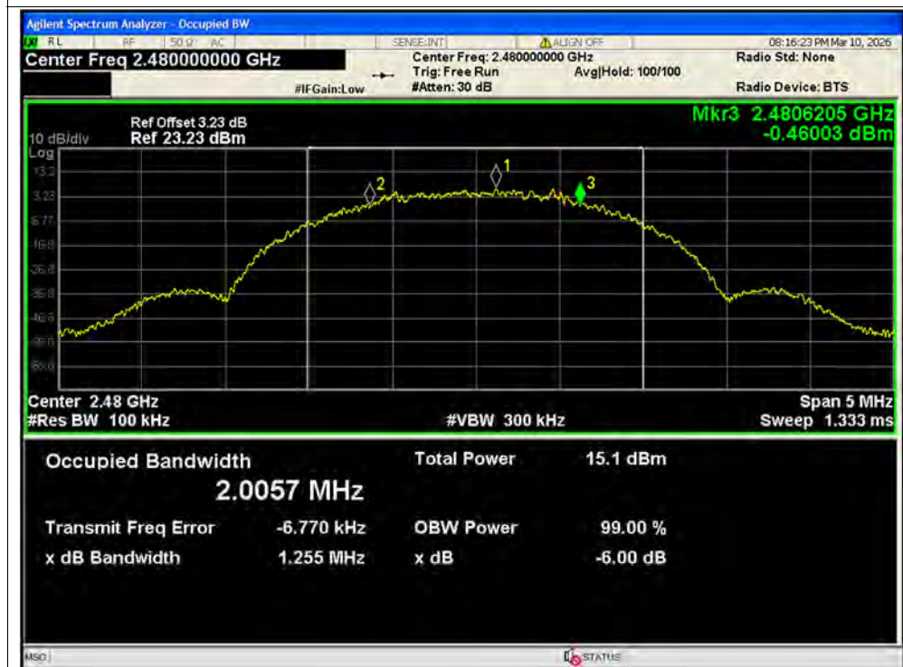
-6dB Bandwidth NVNT BLE 2M 2480MHz Ant2
