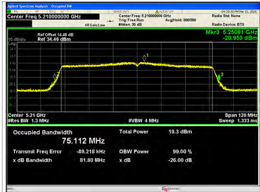
-26dB Bandwidth NVNT ac80 5210MHz Ant1 MIMO
