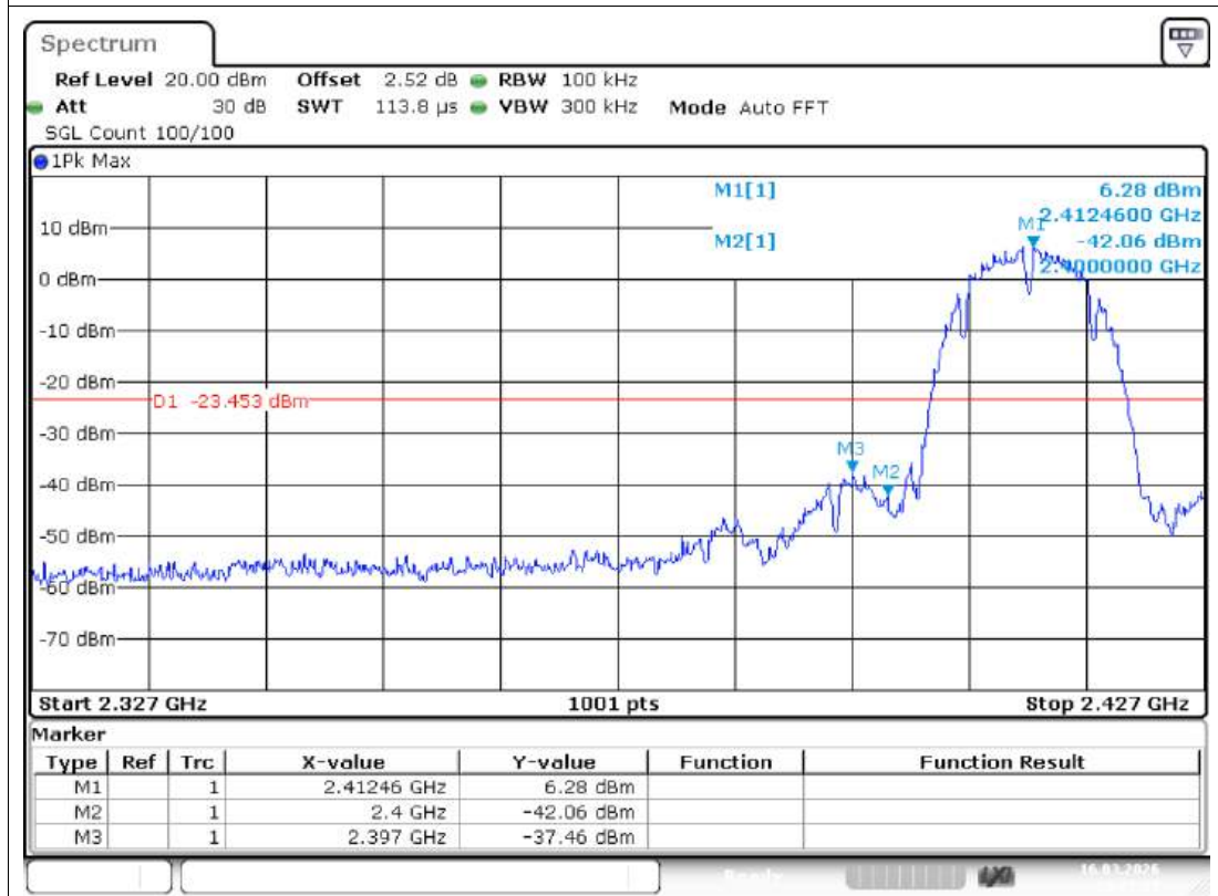
Band Edge NVNT b 2412MHz Ant1 Ref
