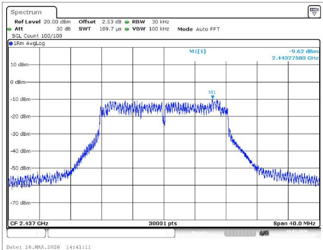
PSD NVNT g 2437MHz Ant1
