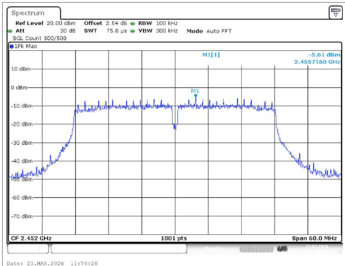
Band Edge NVNT n40 2452MHz Ant1 Ref
