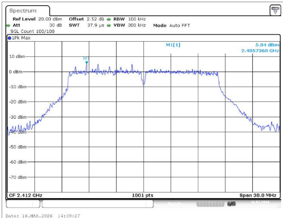
Band Edge NVNT g 2412MHz Ant1 Ref
