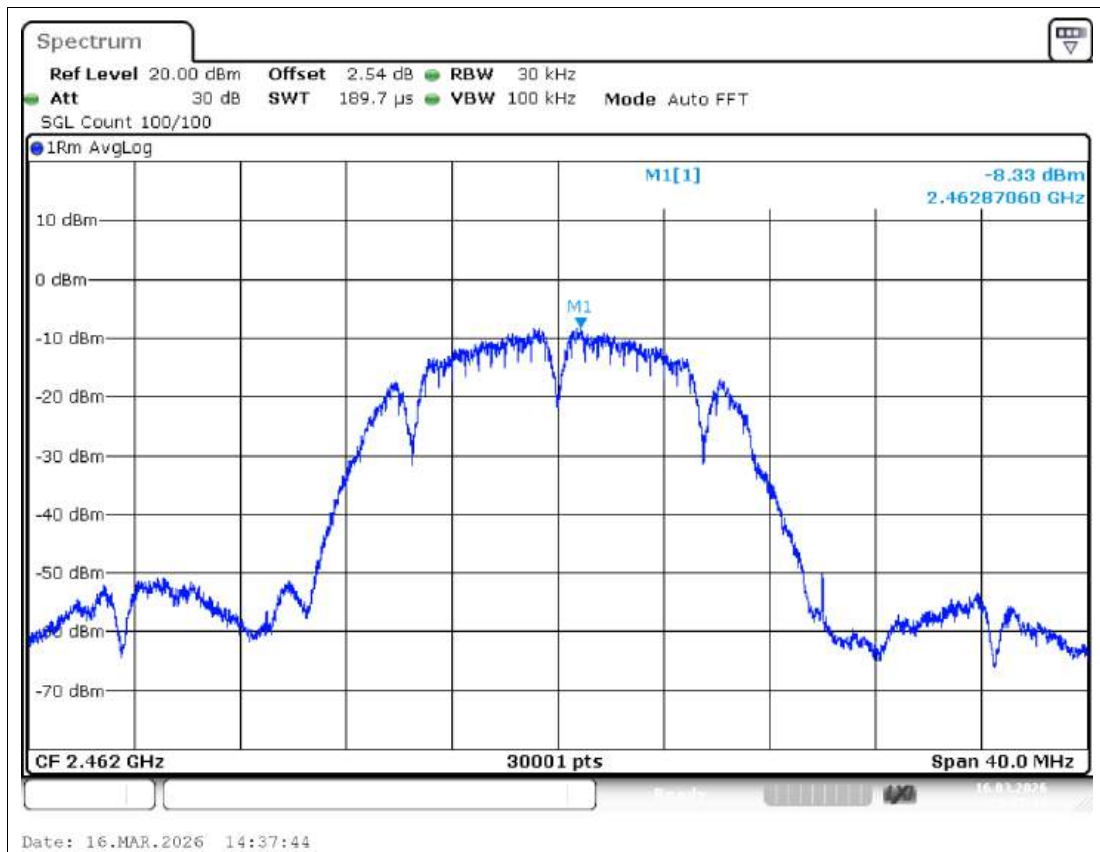
PSD NVNT b 2462MHz Ant1
