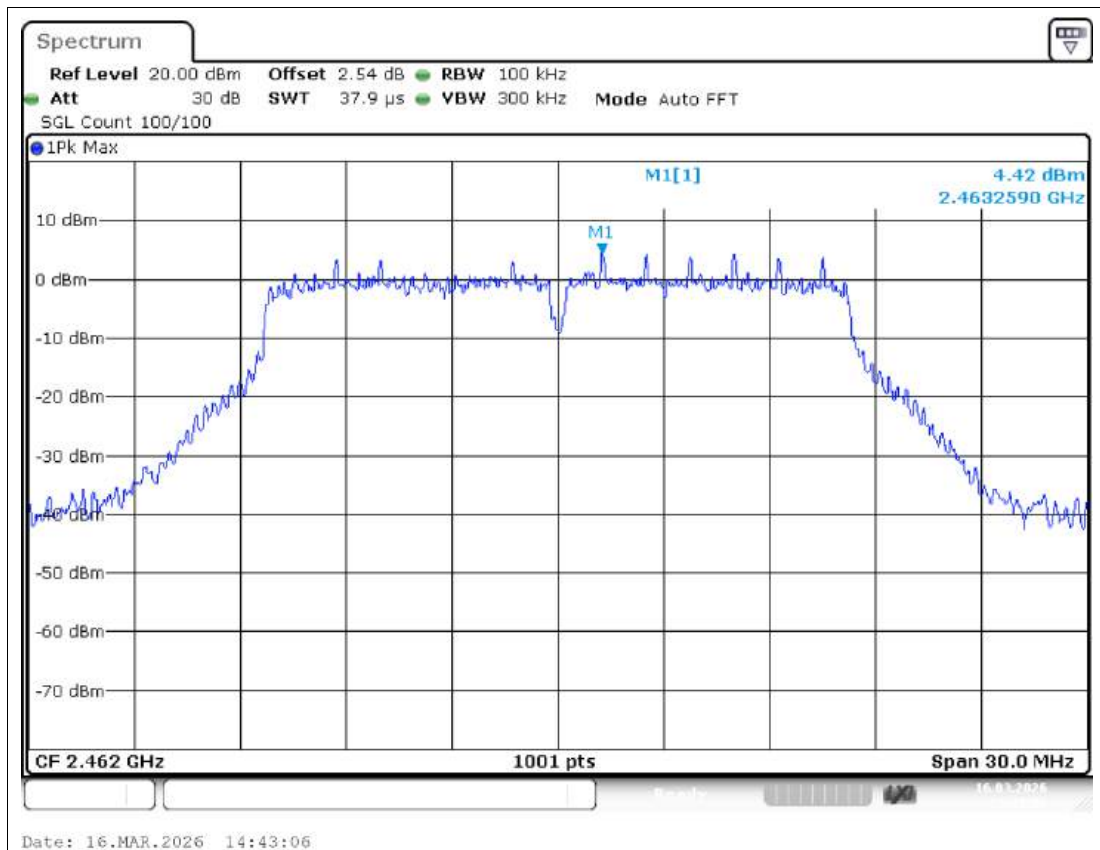
Band Edge NVNT g 2462MHz Ant1 Ref
