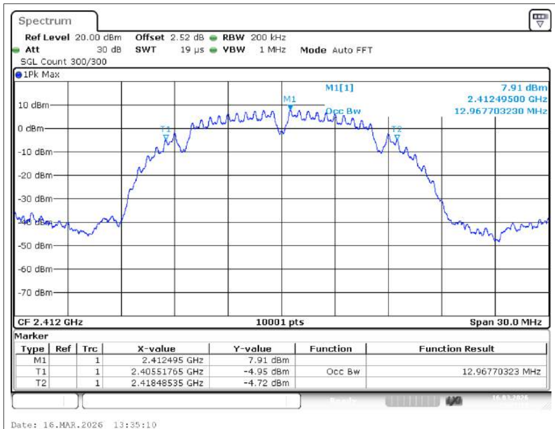
OBW NVNT b 2412MHz Ant1
