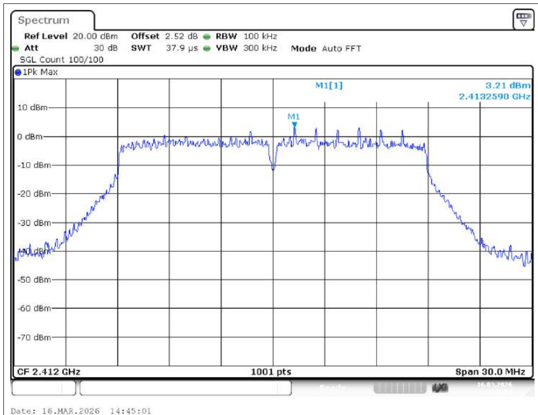
Band Edge NVNT n20 2412MHz Ant1 Ref
