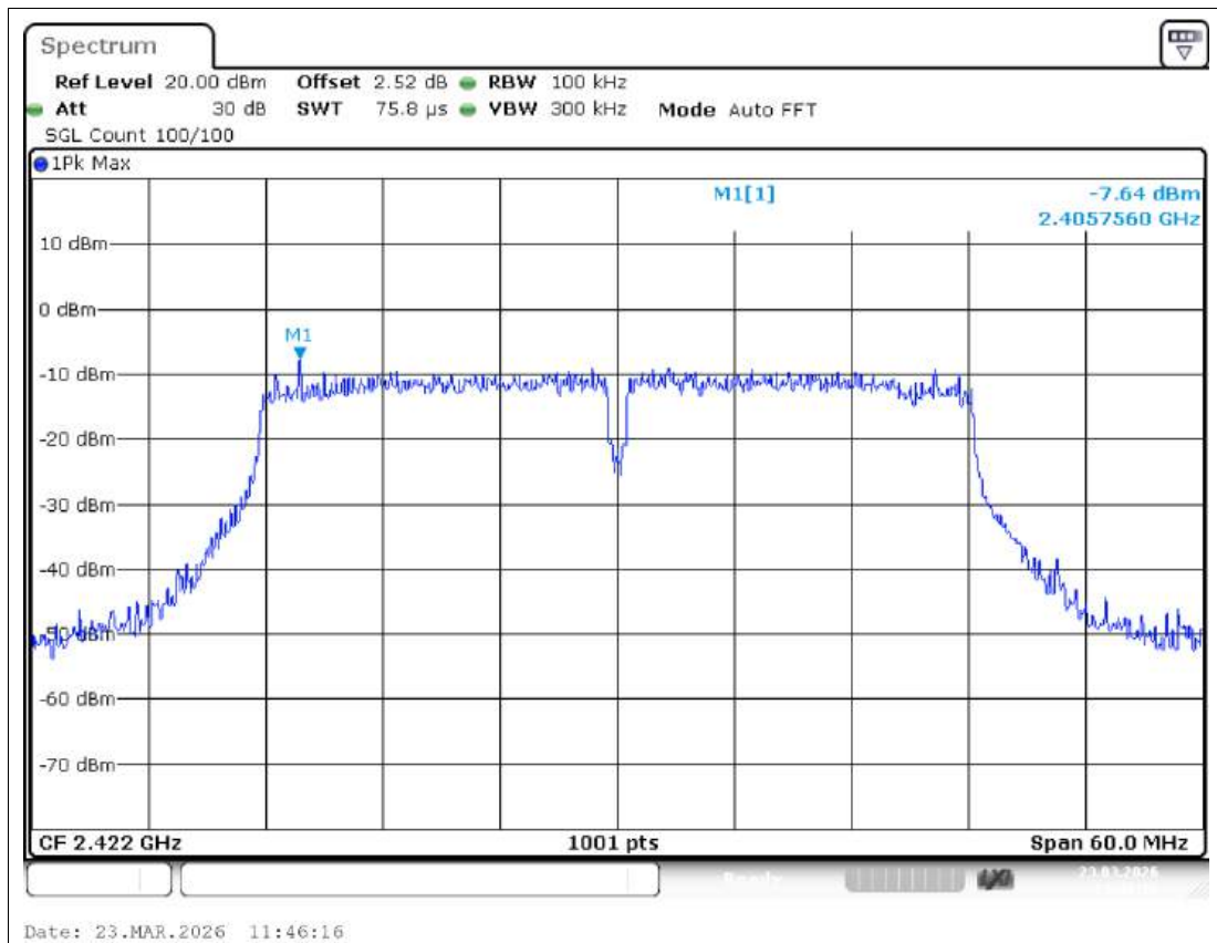
Band Edge NVNT n40 2422MHz Ant1 Ref
