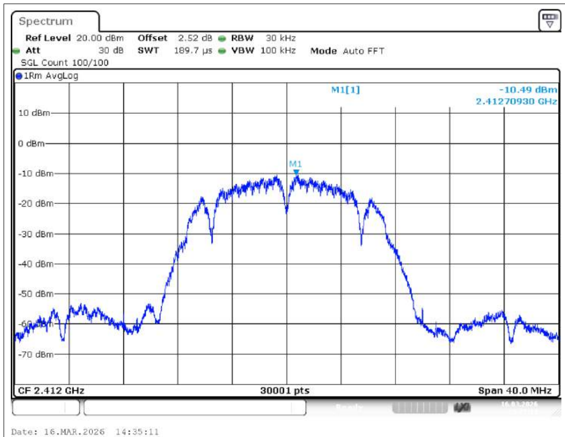
PSD NVNT b 2412MHz Ant1
