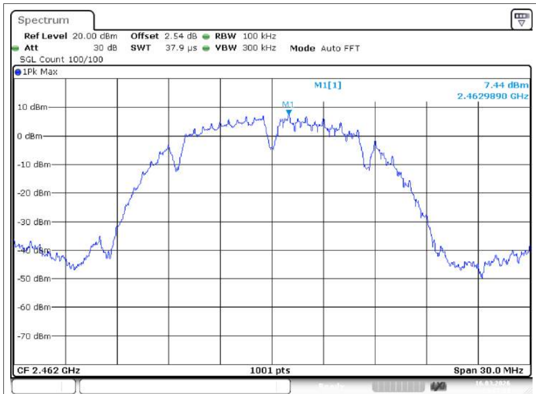
Band Edge NVNT b 2462MHz Ant1 Ref
