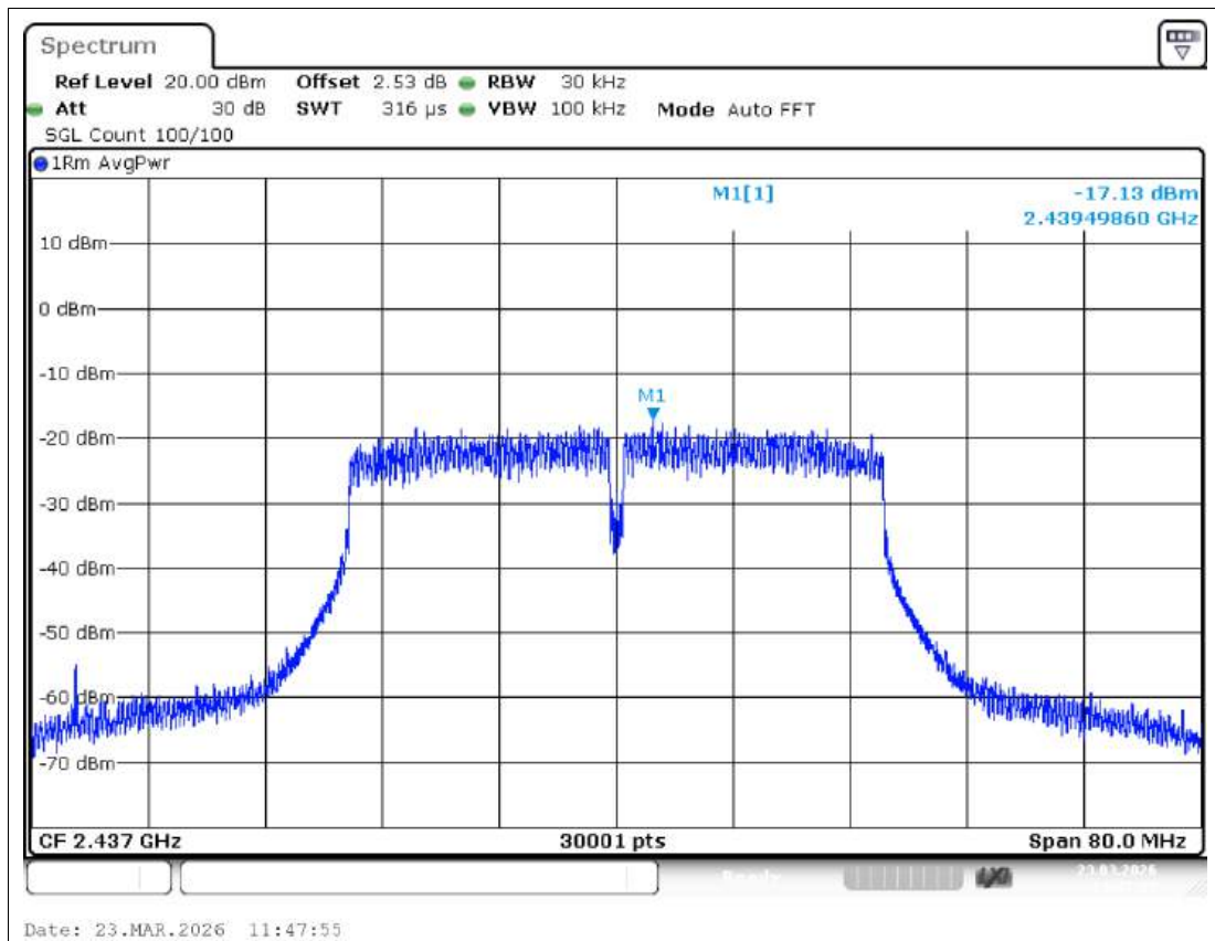
PSD NVNT n40 2437MHz Ant1
