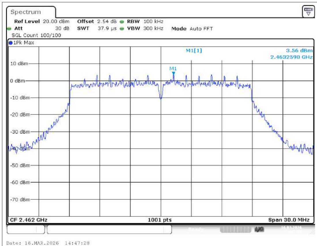
Band Edge NVNT n20 2462MHz Ant1 Ref
