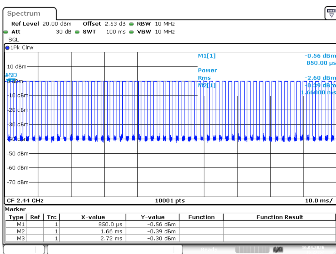
Duty Cycle NVNT BLE 2M 2440MHz Ant1
