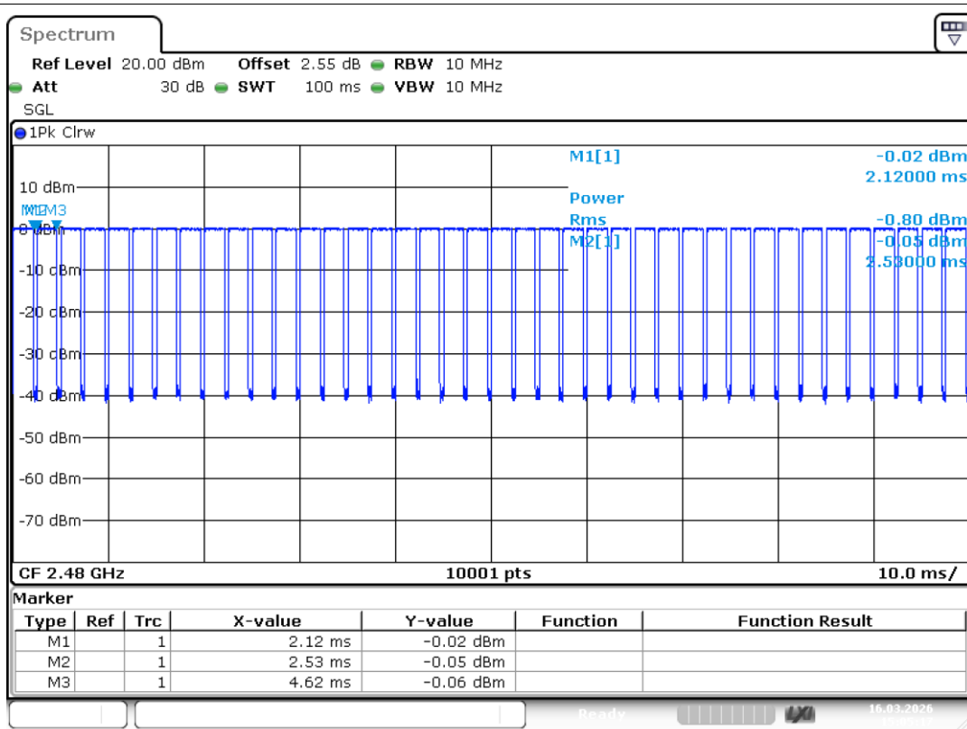
Duty Cycle NVNT BLE 1M 2480MHz Ant1
