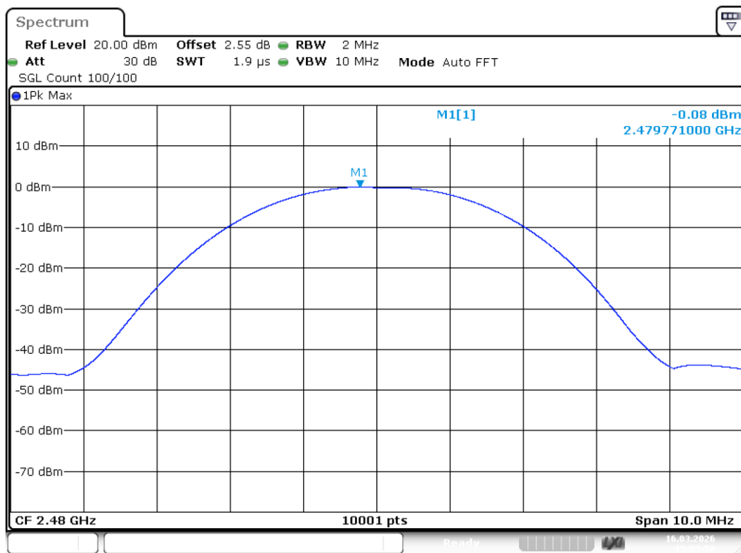
Peak Power NVNT BLE 1M 2480MHz Ant1
