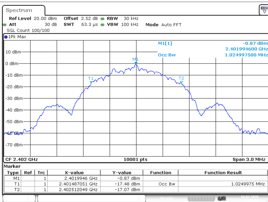
OBW NVNT BLE 1M 2402MHz Ant1
