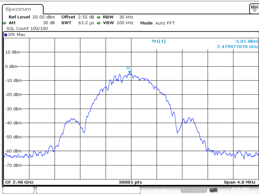
PSD NVNT BLE 1M 2480MHz Ant1
