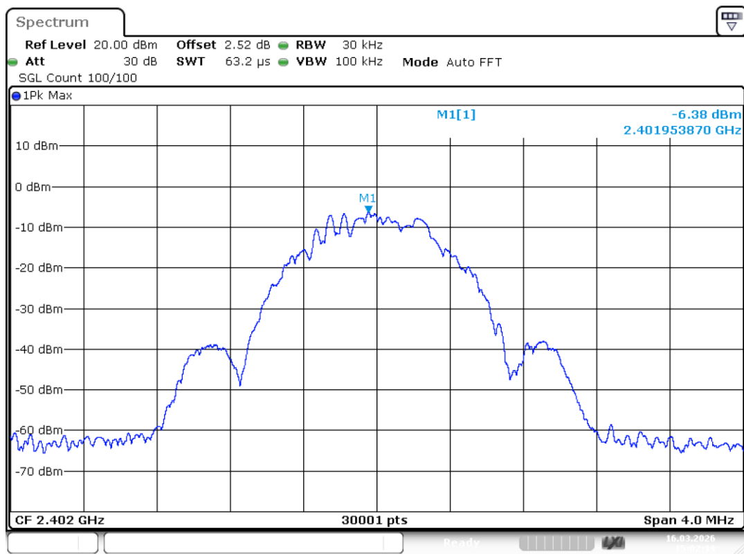
PSD NVNT BLE 1M 2402MHz Ant1
