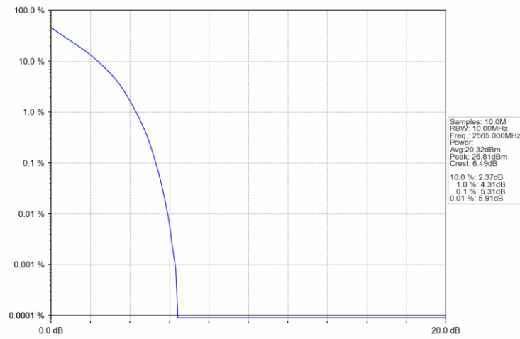
Band7_10MHz_QPSK_HCH_2565MHz_RB_50_0_NTNV
