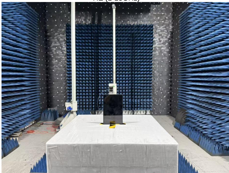
RE (1-18GHz)
