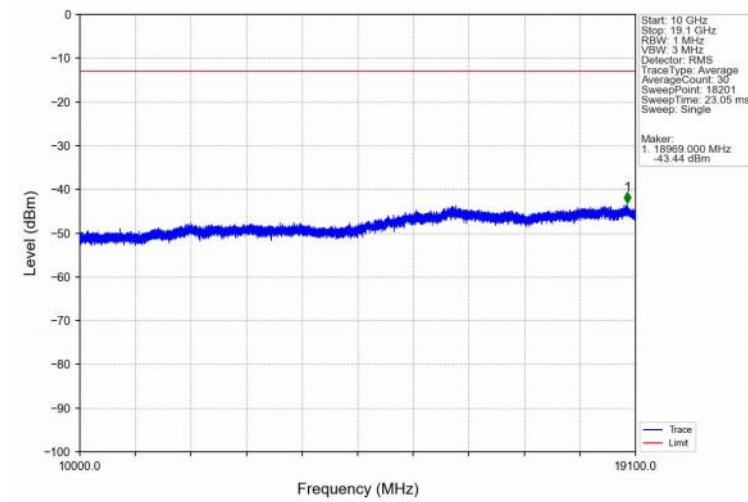
Band2_20MHz_QPSK_LCH_1860MHz_RB_1_0_NTNV
