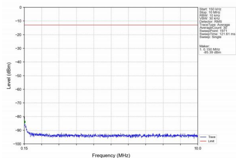
Band2_10MHz_16QAM_HCH_1905MHz_RB_1_0_NTNV
