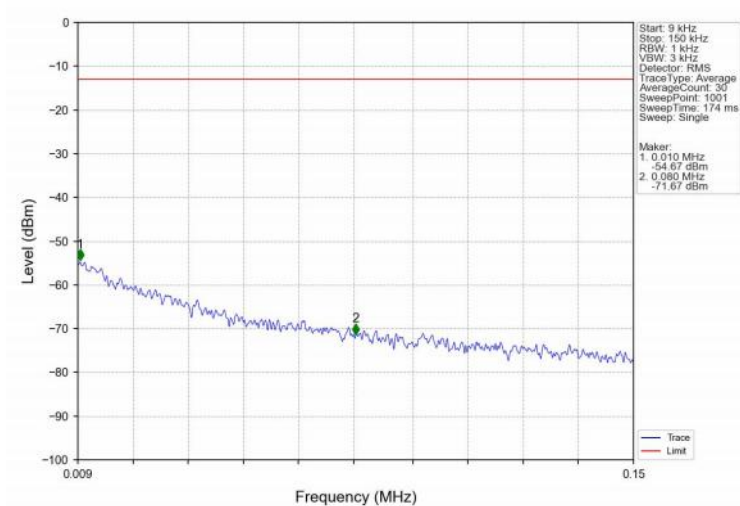
Band2_20MHz_16QAM_HCH_1900MHz_RB_1_0_NTNV
