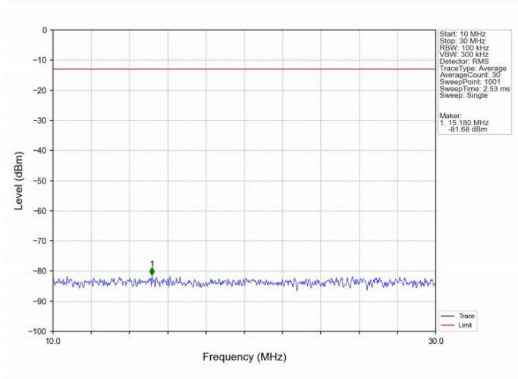
Band2_10MHz_QPSK_MCH_1880MHz_RB_1_0_NTNV
