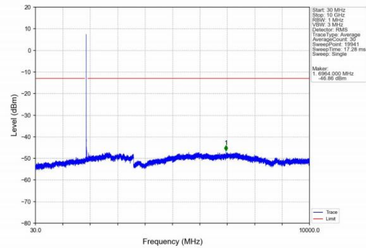
Band2_10MHz_16QAM_MCH_1880MHz_RB_1_0_NTNV
