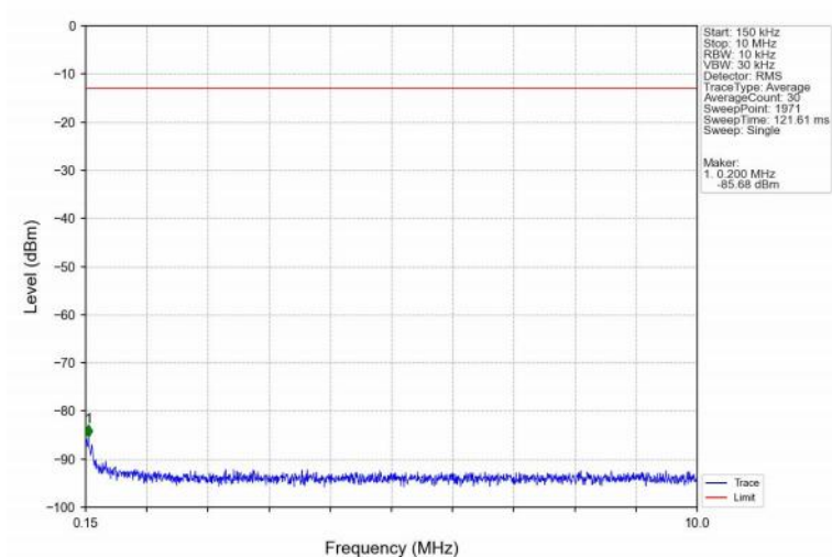
Band2_20MHz_QPSK_MCH_1880MHz_RB_1_0_NTNV
