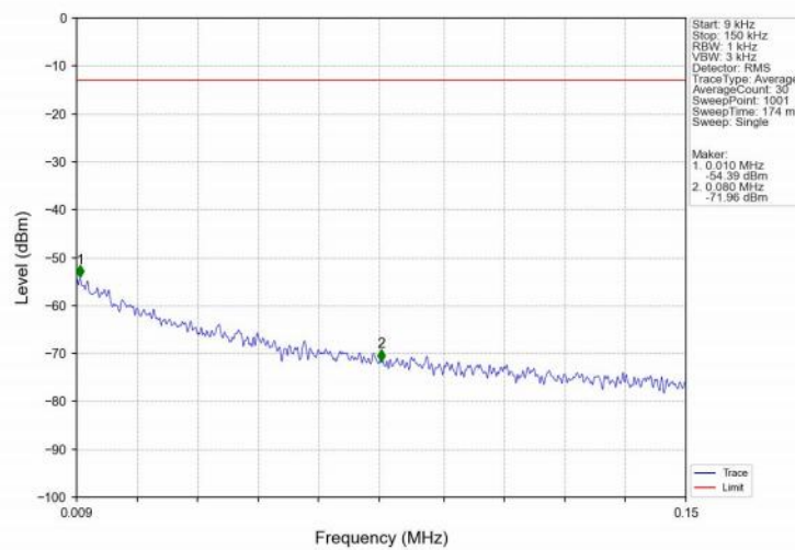
Band2_20MHz_QPSK_LCH_1860MHz_RB_1_0_NTNV
