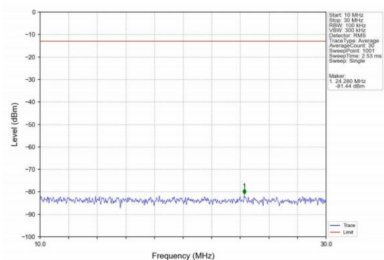
Band2_15MHz_QPSK_HCH_1902.5MHz_RB_1_0_NTNV
