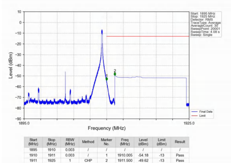
Band2_15MHz_QPSK_HCH_1902.5MHz_RB_1_74_NTNV
