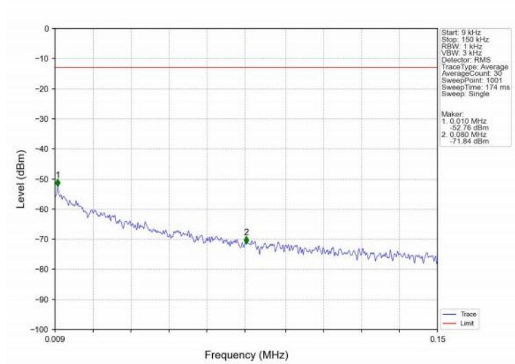
Band2_15MHz_QPSK_HCH_1902.5MHz_RB_1_0_NTNV
