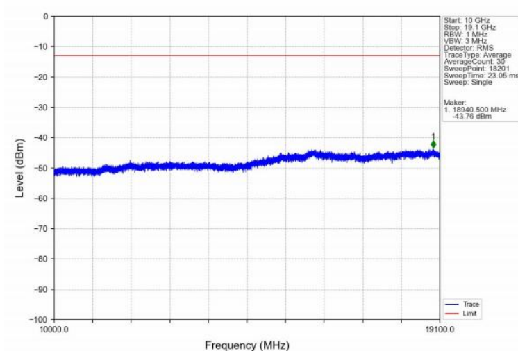
Band2_10MHz_16QAM_HCH_1905MHz_RB_1_0_NTNV
