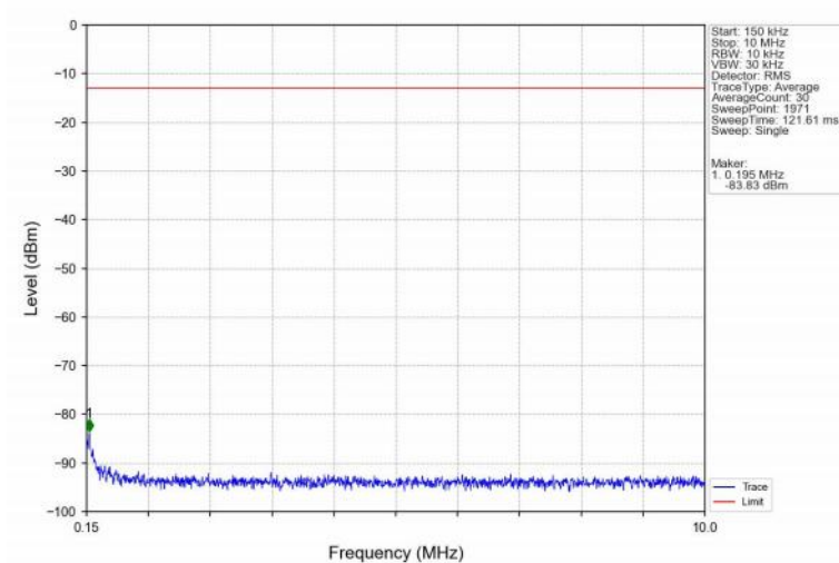
Band2_20MHz_QPSK_HCH_1900MHz_RB_1_0_NTNV
