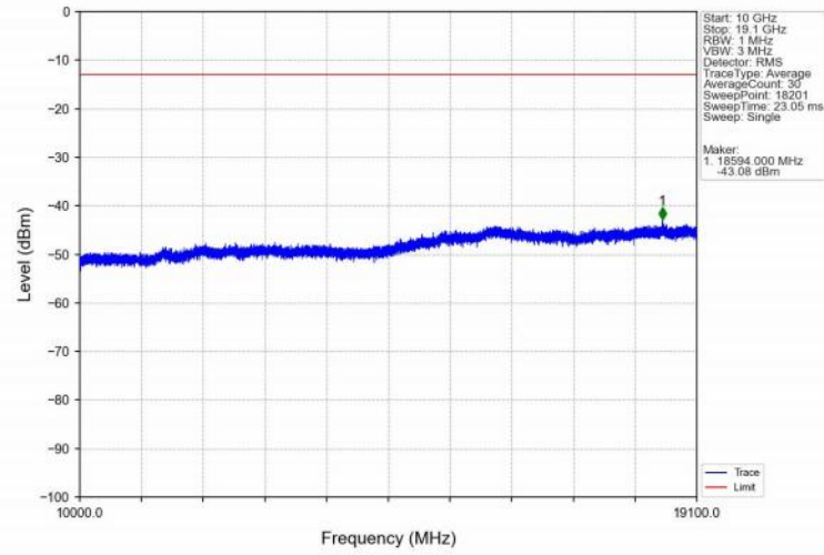
Band2_10MHz_QPSK_HCH_1905MHz_RB_1_49_NTNV
