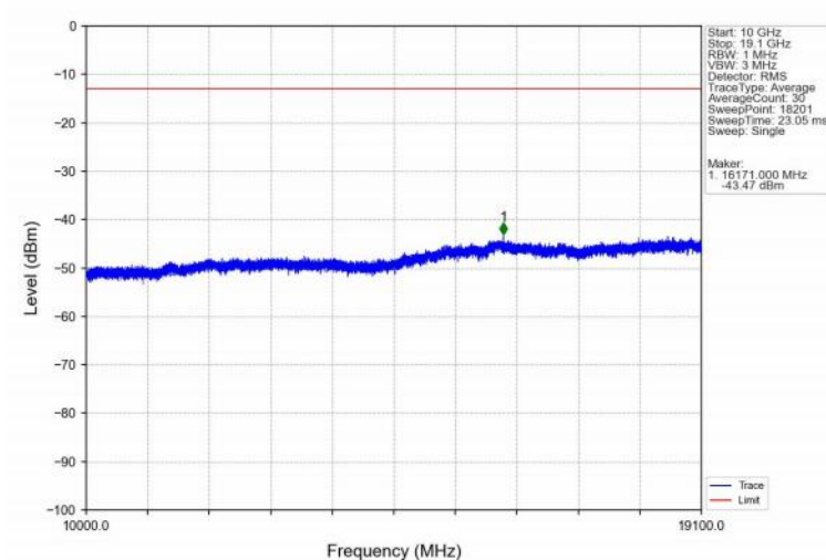
Band2_20MHz_16QAM_HCH_1900MHz_RB_1_0_NTNV
