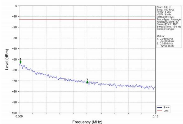
Band2_20MHz_QPSK_HCH_1900MHz_RB_1_0_NTNV
