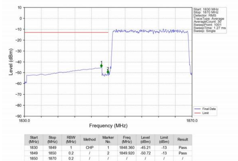
Band2_20MHz_16QAM_LCH_1860MHz_RB_100_0_NTNV
