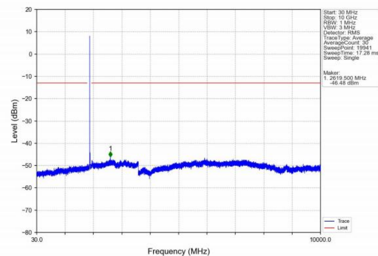
Band2_20MHz_QPSK_HCH_1900MHz_RB_1_0_NTNV
