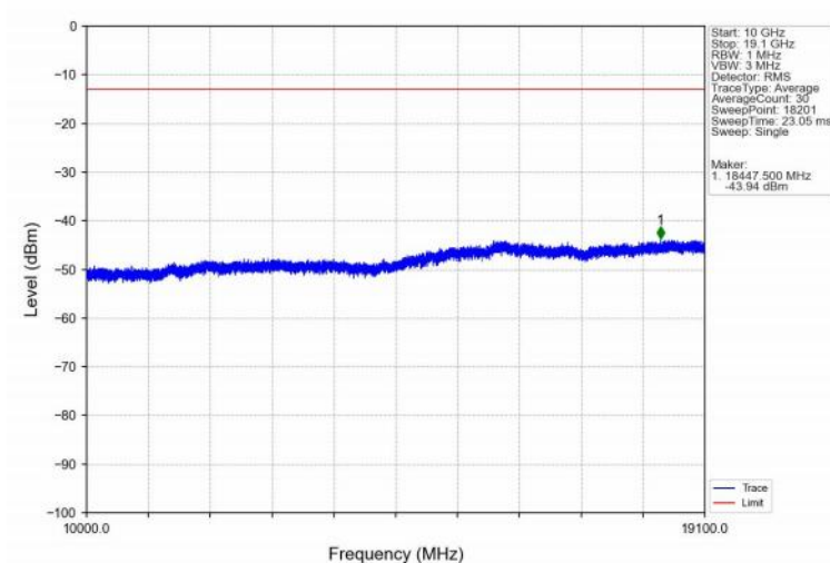
Band2_10MHz_16QAM_LCH_1855MHz_RB_50_0_NTNV
