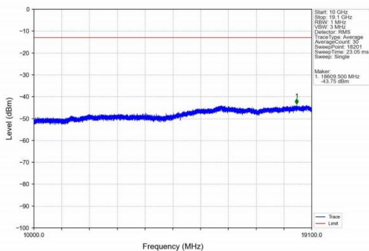
Band2_20MHz_QPSK_MCH_1880MHz_RB_1_0_NTNV
