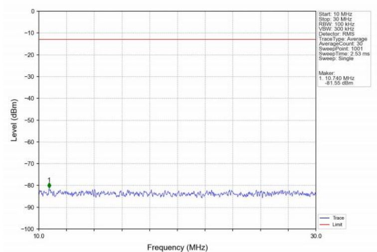
Band2_15MHz_QPSK_LCH_1857.5MHz_RB_1_0_NTNV
