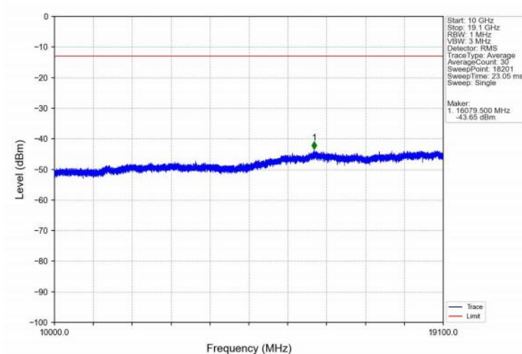
Band2_15MHz_QPSK_HCH_1902.5MHz_RB_1_74_NTNV
