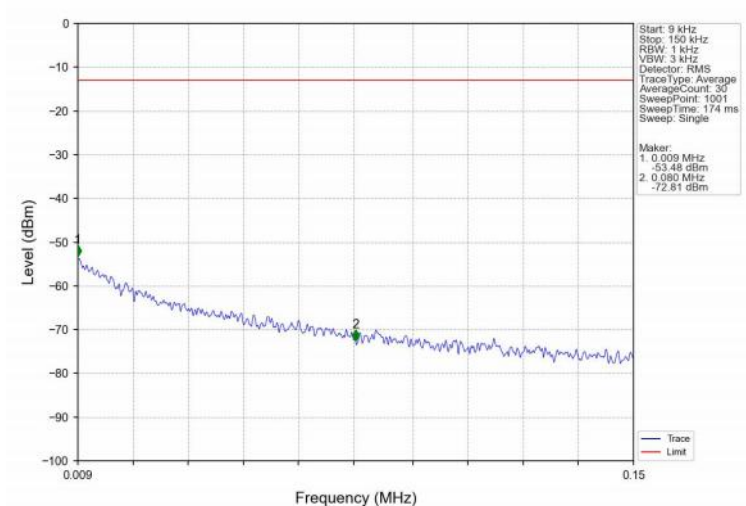
Band2_10MHz_16QAM_LCH_1855MHz_RB_1_0_NTNV
