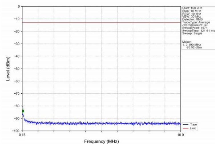
Band2_10MHz_16QAM_LCH_1855MHz_RB_1_0_NTNV
