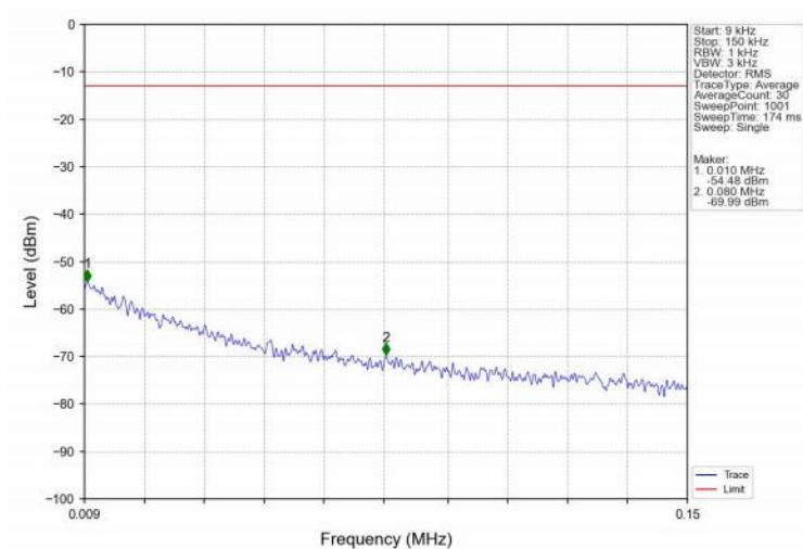
Band2_10MHz_16QAM_HCH_1905MHz_RB_1_0_NTNV
