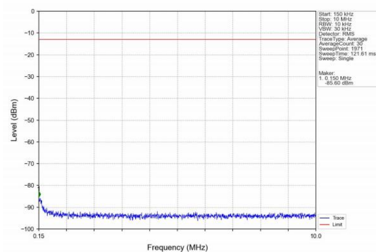
Band2_10MHz_16QAM_MCH_1880MHz_RB_1_0_NTNV
