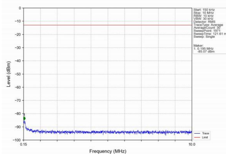
Band2_20MHz_16QAM_LCH_1860MHz_RB_1_0_NTNV
