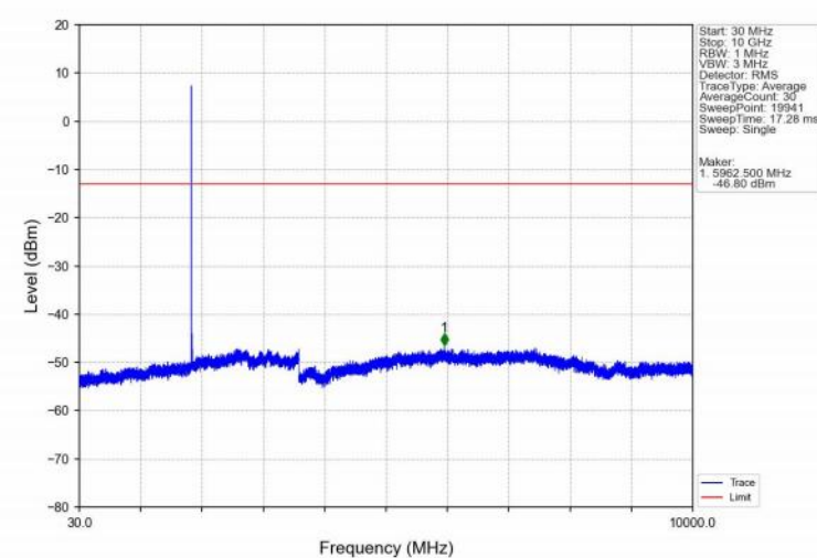
Band2_10MHz_16QAM_LCH_1855MHz_RB_1_0_NTNV
