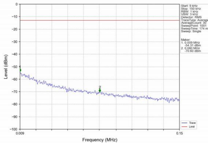
Band2_15MHz_QPSK_LCH_1857.5MHz_RB_1_0_NTNV
