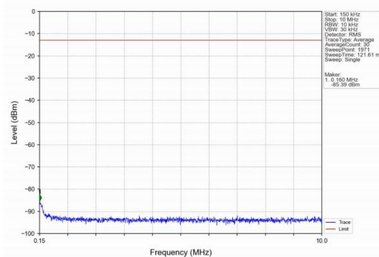
Band2_10MHz_QPSK_HCH_1905MHz_RB_1_0_NTNV
