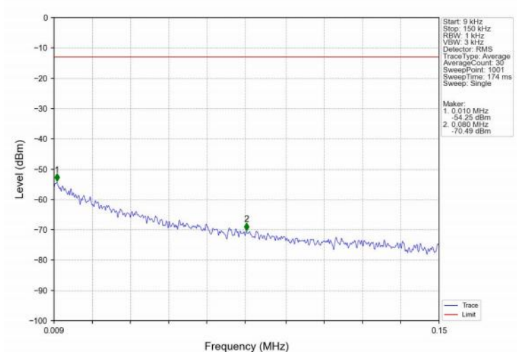
Band2_20MHz_16QAM_LCH_1860MHz_RB_1_0_NTNV
