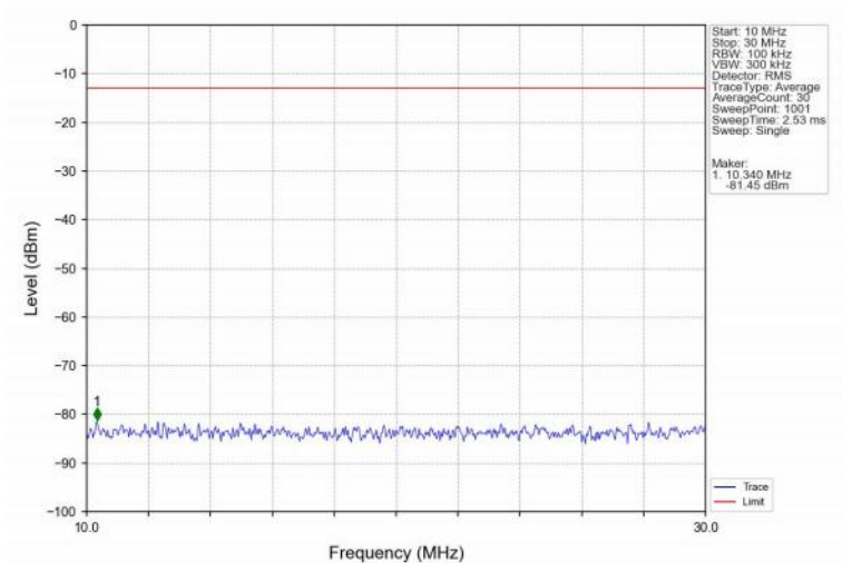
Band2_20MHz_QPSK_LCH_1860MHz_RB_1_0_NTNV
