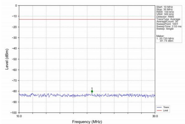
Band2_15MHz_QPSK_MCH_1880MHz_RB_1_0_NTNV
