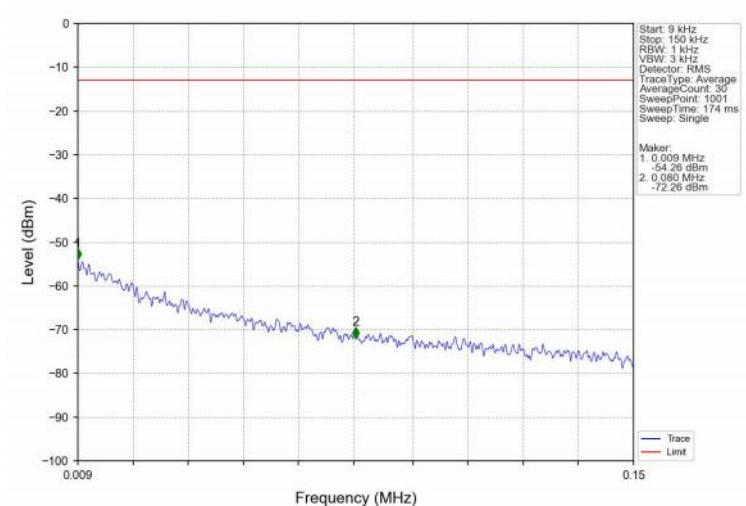
Band2_10MHz_16QAM_MCH_1880MHz_RB_1_0_NTNV
