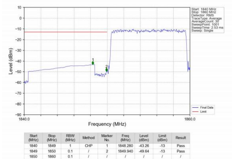
Band2_10MHz_16QAM_LCH_1855MHz_RB_50_0_NTNV
