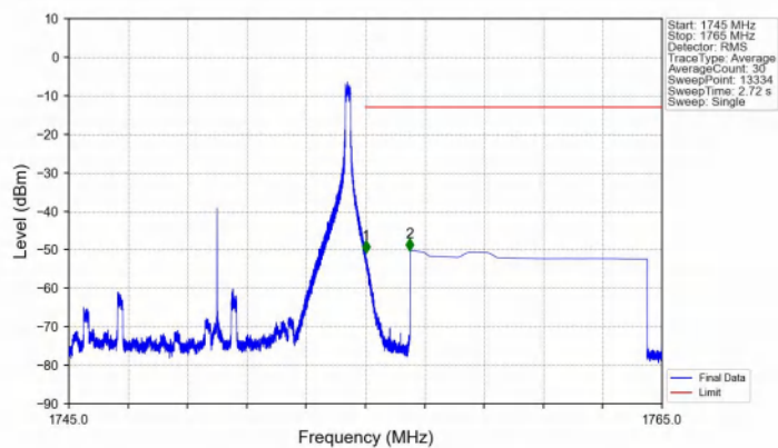
Band4_10MHz_QPSK_HCH_1750MHz_RB_1_49_NTNV
