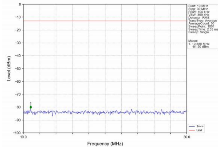
Band4_20MHz_QPSK_LCH_1720MHz_RB_1_0_NTNV
