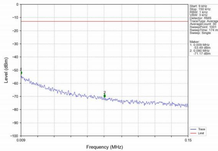
Band4_15MHz_QPSK_LCH_1717.5MHz_RB_1_0_NTNV
