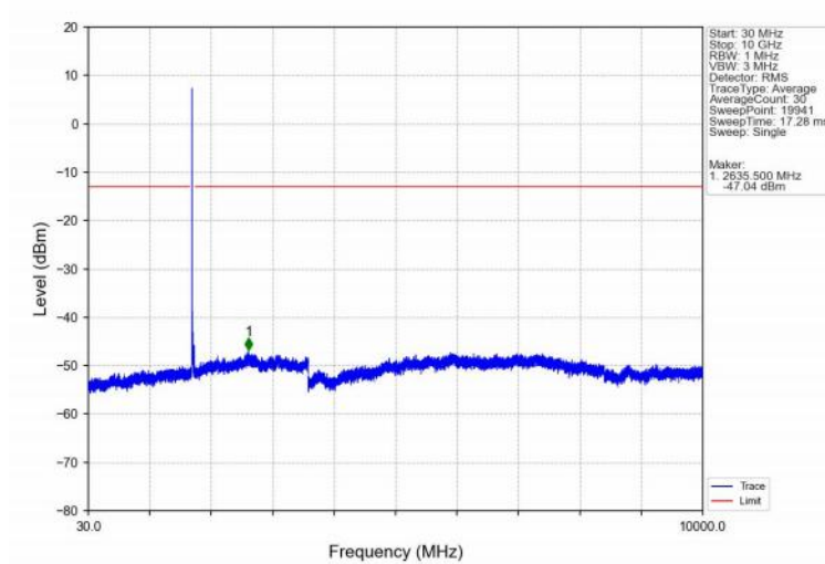
Band4_20MHz_16QAM_LCH_1720MHz_RB_1_0_NTNV
