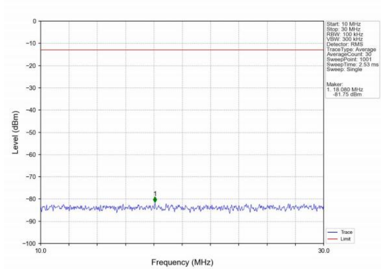
Band4_20MHz_QPSK_HCH_1745MHz_RB_1_0_NTNV
