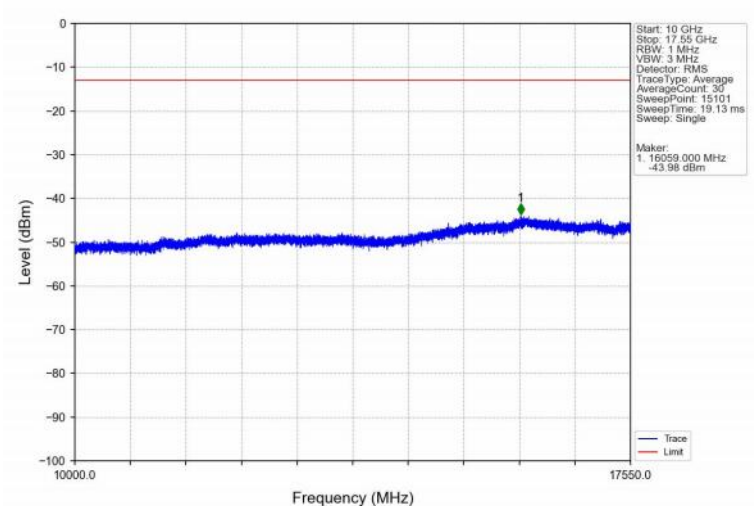
Band4_10MHz_QPSK_HCH_1750MHz_RB_1_49_NTNV
