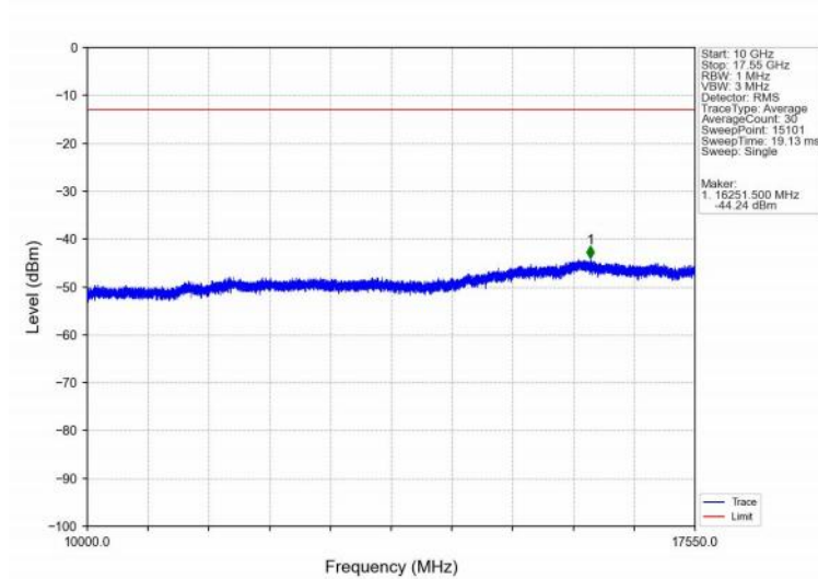
Band4_20MHz_QPSK_LCH_1720MHz_RB_1_0_NTNV
