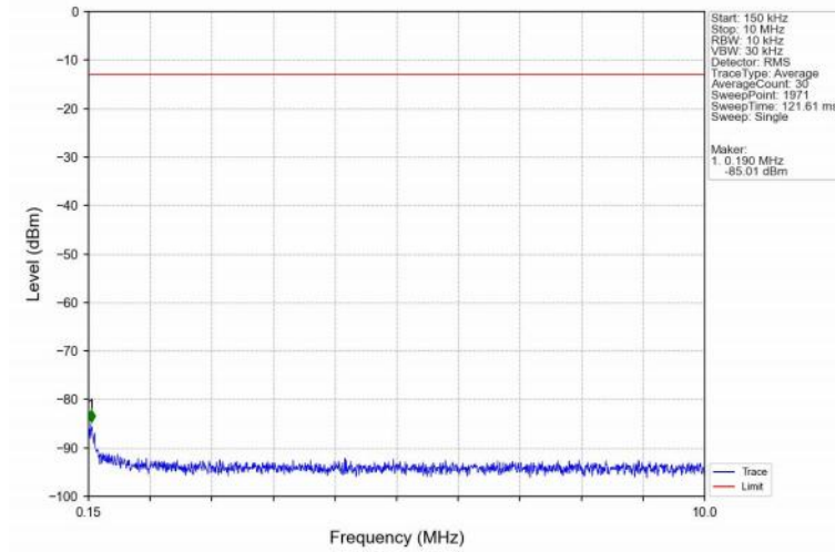
Band4_20MHz_QPSK_LCH_1720MHz_RB_1_0_NTNV
