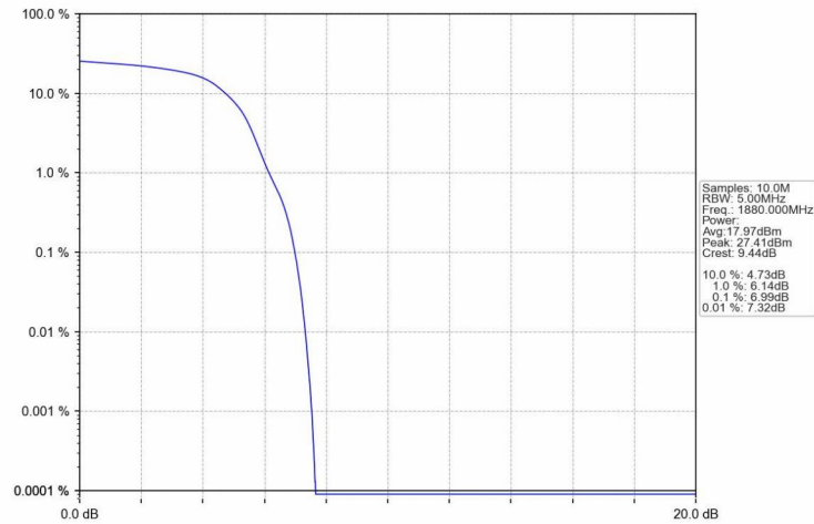
Band2_HSUPA_MCH_1880MHz_Subtest 1_NTNV
