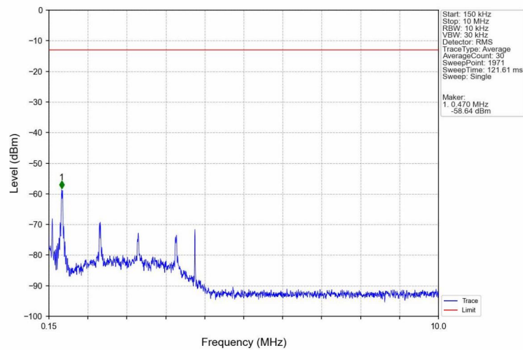
Band2_HSUPA_MCH_1880MHz_Subtest 1_NTNV
