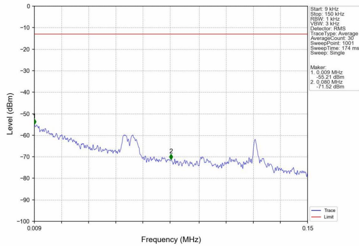
Band4_HSUPA_LCH_1712.4MHz_Subtest 1_NTNV
