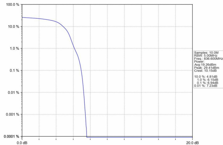
Band5_HSUPA_MCH_836.6MHz_Subtest 1_NTNV
