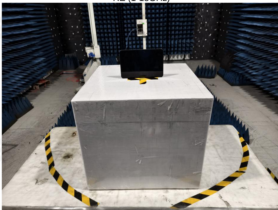
RE (1-18GHz)
