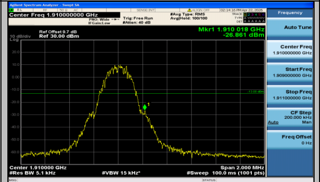
GPRS1900-810-0-PASS
