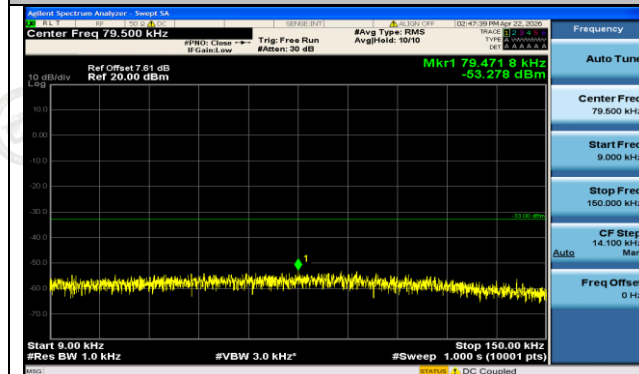
GSM850-190-5-0.009~0.15MHz-PASS
