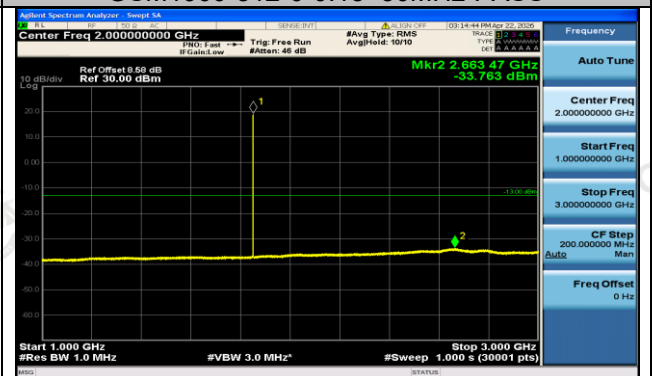
GSM1900-512-0-1000~3000MHz-PASS
