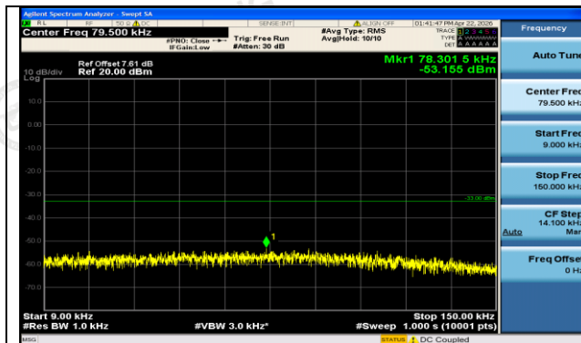
GPRS850-128-5-0.009~0.15MHz-PASS
