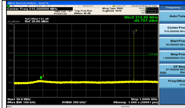
EGPRS850-190-8-30~1000MHz-PASS
