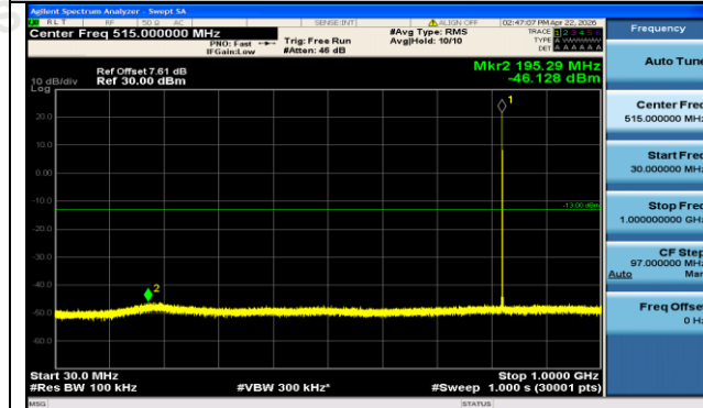
GSM850-128-5-30~1000MHz-PASS
