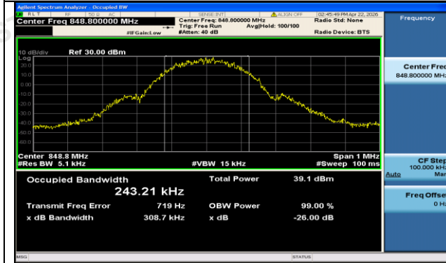
GSM850-251-5-PASS
