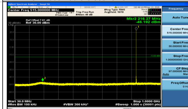
GSM850-190-5-30~1000MHz-PASS
