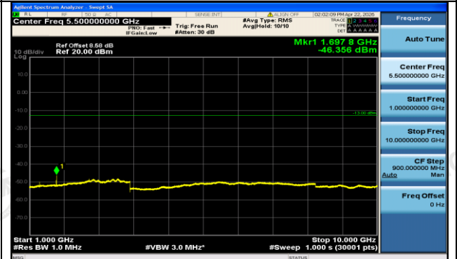
EGPRS850-251-8-1000~10000MHz-PASS
