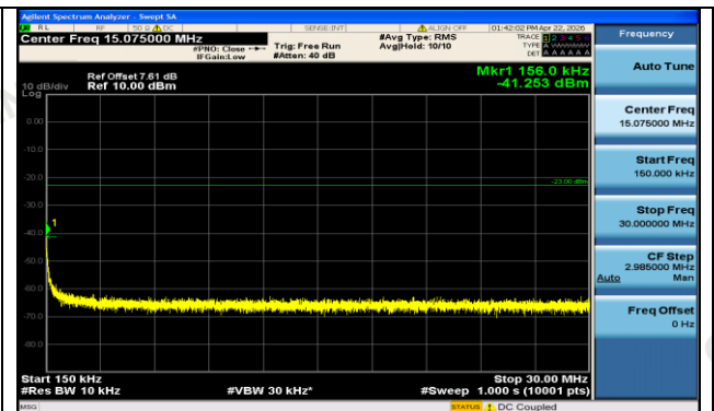
GPRS850-128-5-0.15~30MHz-PASS
