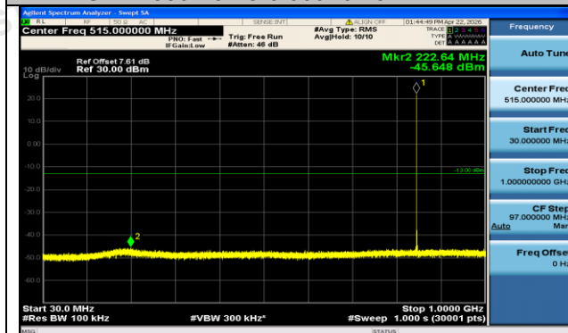
GPRS850-251-5-30~1000MHz-PASS
