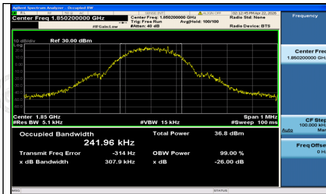
GPRS1900-512-0-PASS
