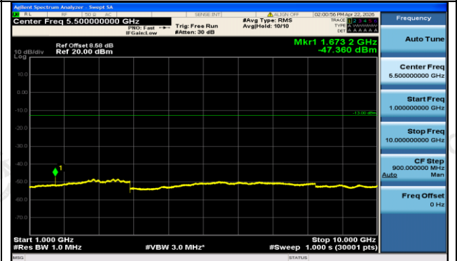
EGPRS850-190-8-1000~10000MHz-PASS
