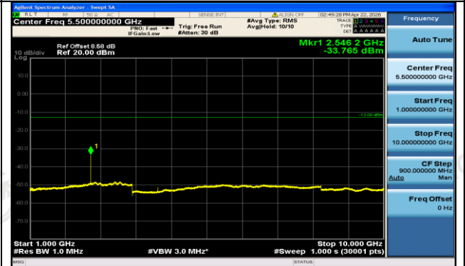
GSM850-251-5-1000~10000MHz-PASS
