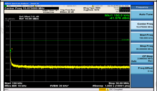
GPRS850-251-5-0.15~30MHz-PASS
