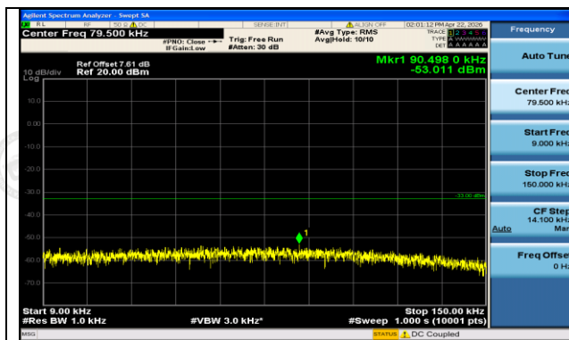
EGPRS850-251-8-0.009~0.15MHz-PASS
