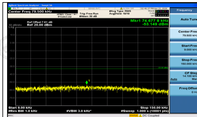
GSM850-128-5-0.009~0.15MHz-PASS
