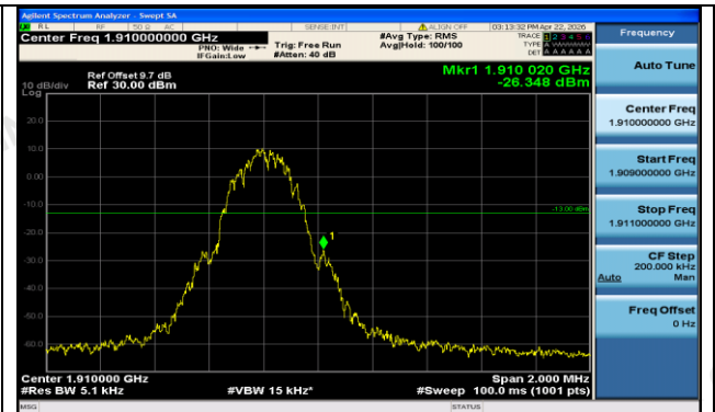
GSM1900-810-0-PASS
