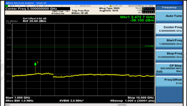
GSM850-128-5-1000~10000MHz-PASS
