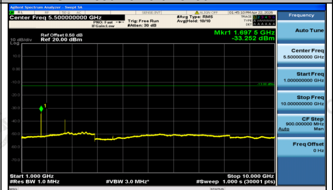
GPRS850-251-5-1000~10000MHz-PASS
