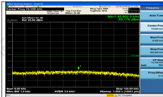
GSM850-251-5-0.009~0.15MHz-PASS
