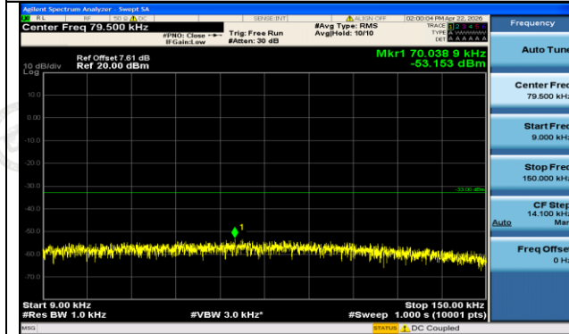
EGPRS850-190-8-0.009~0.15MHz-PASS
