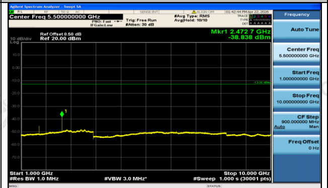
GPRS850-128-5-1000~10000MHz-PASS
