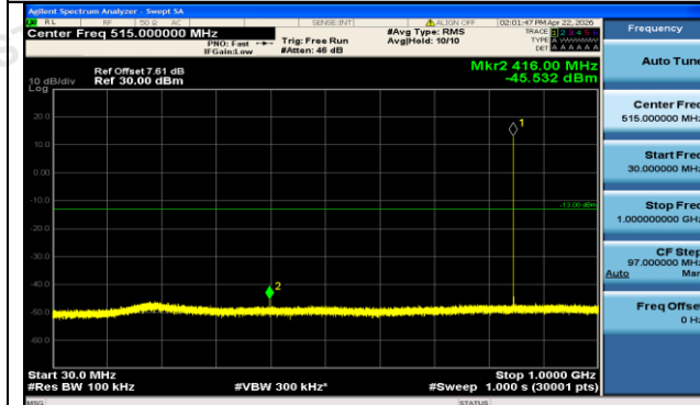
EGPRS850-251-8-30~1000MHz-PASS
