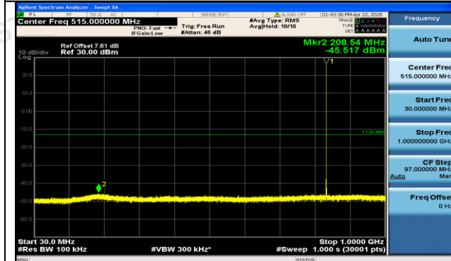
GPRS850-190-5-30~1000MHz-PASS
