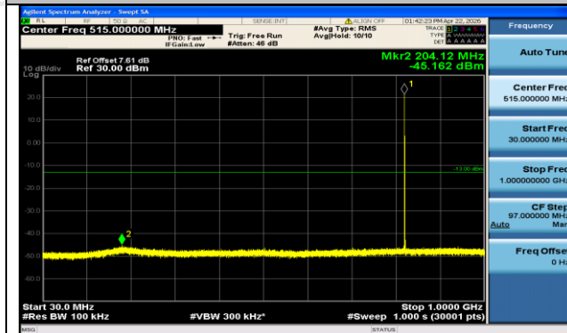
GPRS850-128-5-30~1000MHz-PASS
