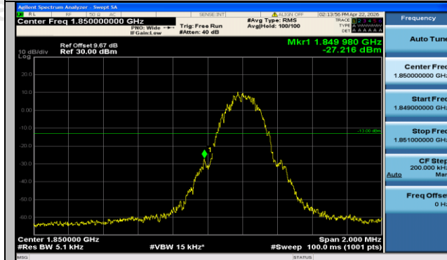
GPRS1900-512-0-PASS
