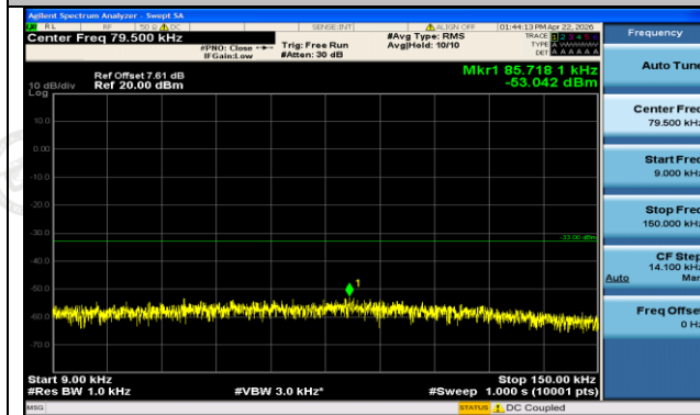
GPRS850-251-5-0.009~0.15MHz-PASS
