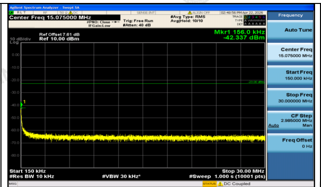
GSM850-251-5-0.15~30MHz-PASS
