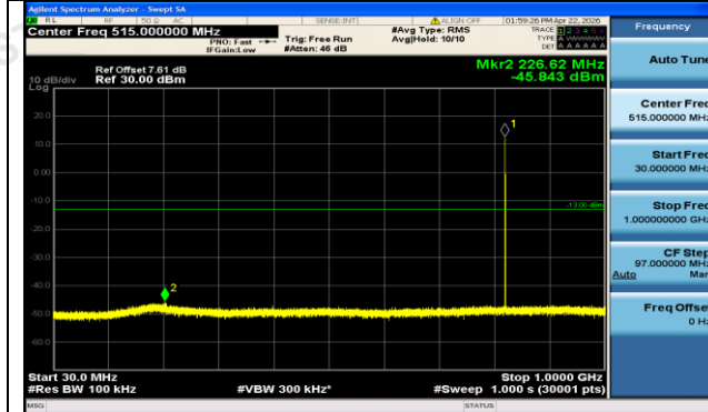
EGPRS850-128-8-30~1000MHz-PASS
