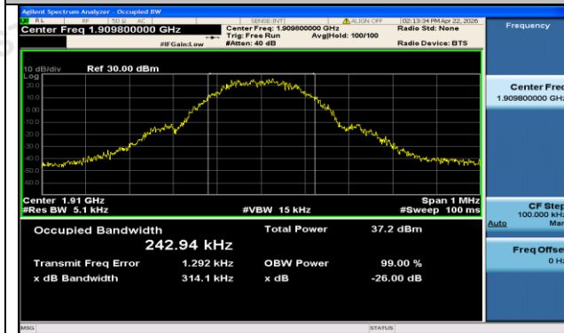
GPRS1900-810-0-PASS
