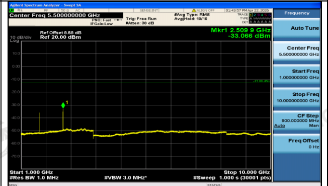
GPRS850-190-5-1000~10000MHz-PASS
