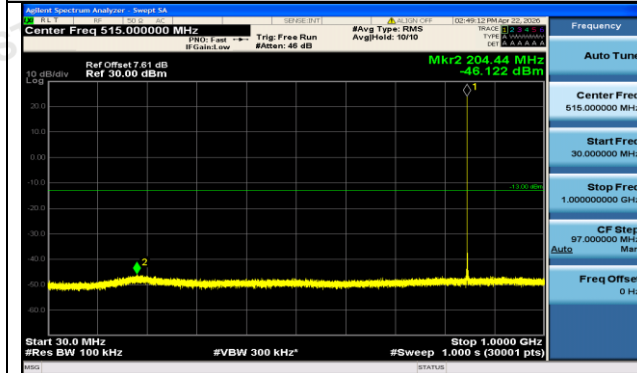
GSM850-251-5-30~1000MHz-PASS
