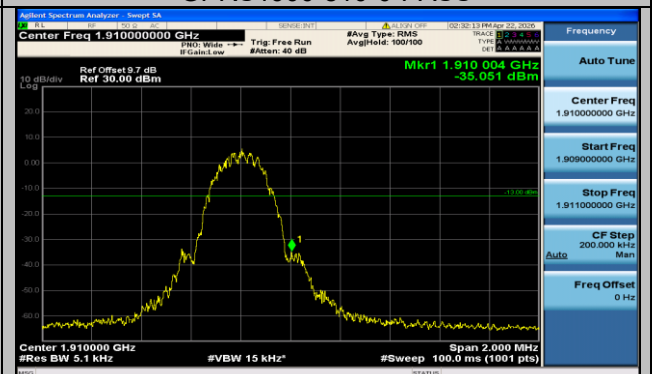
EGPRS1900-810-2-PASS
