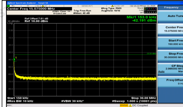
GPRS1900-661-0-0.15~30MHz-PASS
