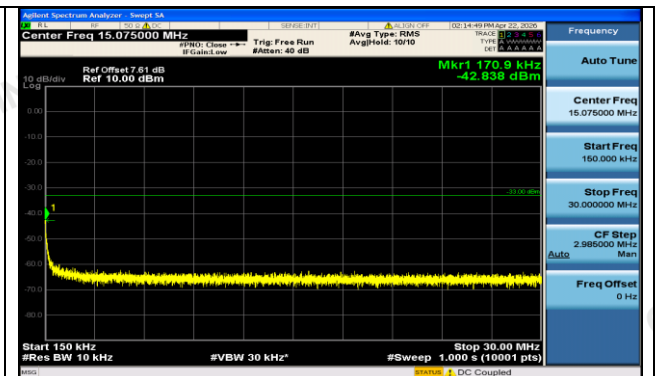
GPRS1900-512-0-0.15~30MHz-PASS
