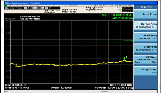
GPRS1900-661-0-3000~18000MHz-PASS
