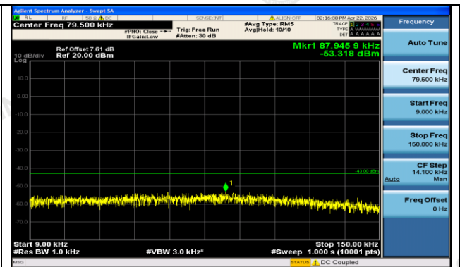
GPRS1900-661-0-0.009~0.15MHz-PASS
