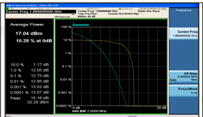
EGPRS1900-661-2-PASS
