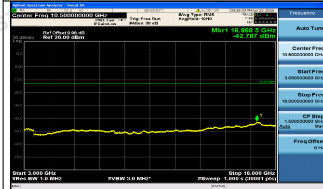
GSM1900-810-0-3000~18000MHz-PASS
