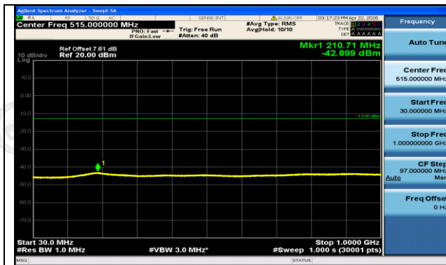
GSM1900-810-0-30~1000MHz-PASS
