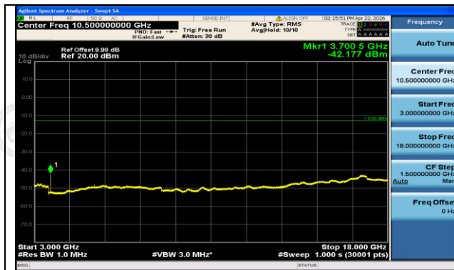
GPRS1900-512-0-3000~18000MHz-PASS
