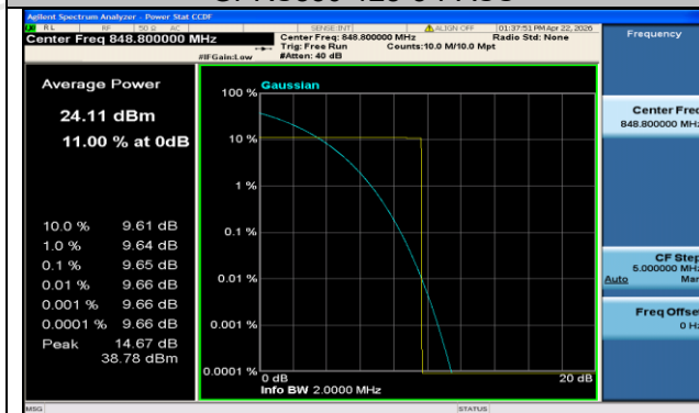
GPRS850-251-5-PASS
