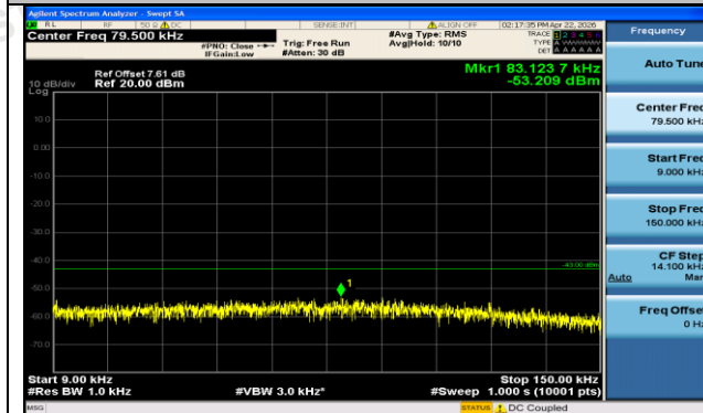
GPRS1900-810-0-0.009~0.15MHz-PASS
