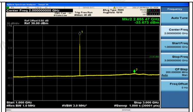
GSM1900-810-0-1000~3000MHz-PASS
