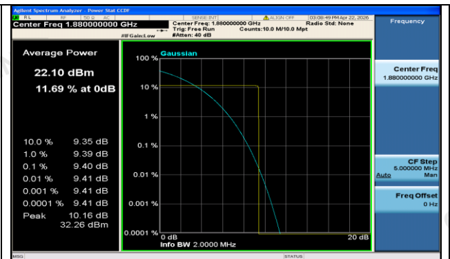
GSM1900-661-0-PASS
