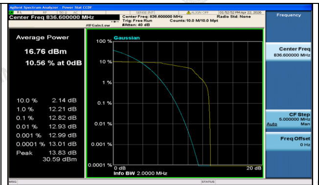
EGPRS850-190-8-PASS
