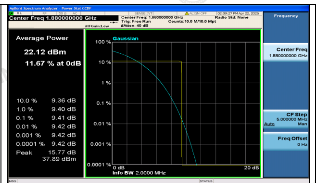
GPRS1900-661-0-PASS
