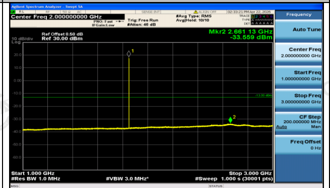
EGPRS1900-512-2-1000~3000MHz-PASS
