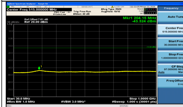
EGPRS1900-512-2-30~1000MHz-PASS
