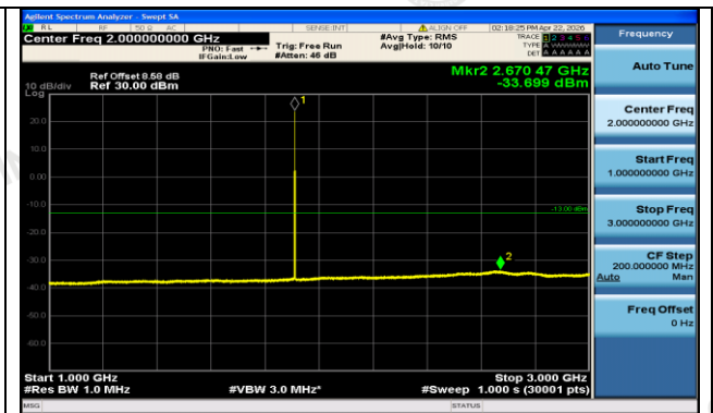
GPRS1900-810-0-1000~3000MHz-PASS
