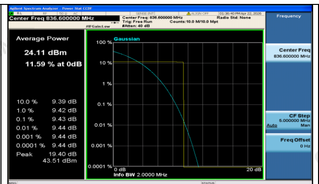
GPRS850-190-5-PASS
