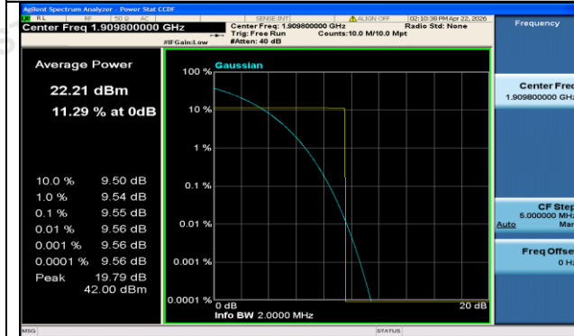
GPRS1900-810-0-PASS
