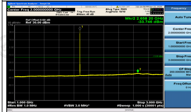
GPRS1900-661-0-1000~3000MHz-PASS
