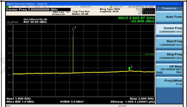
GPRS1900-512-0-1000~3000MHz-PASS
