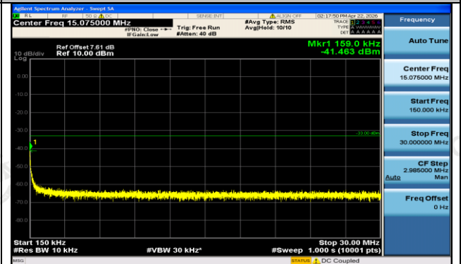
GPRS1900-810-0-0.15~30MHz-PASS
