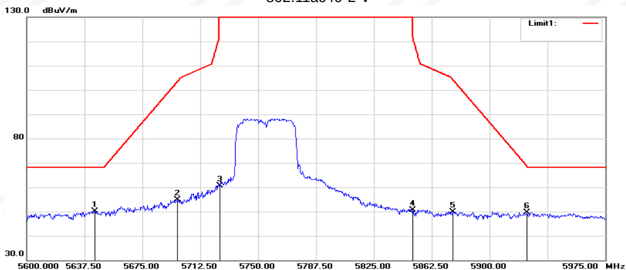
802.11ac40-L-V
