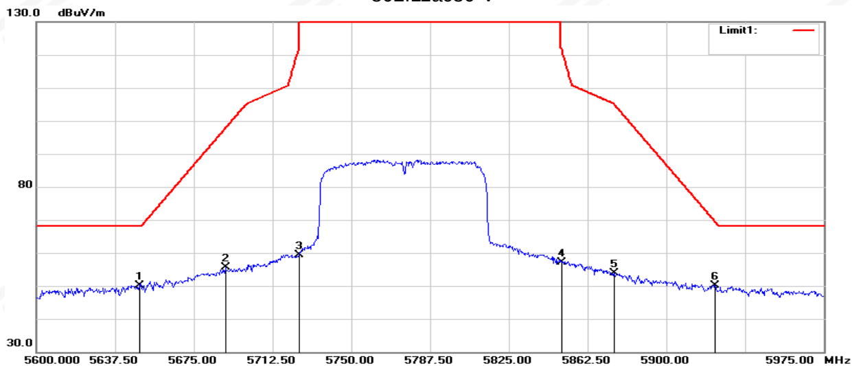
802.11ac80-V
