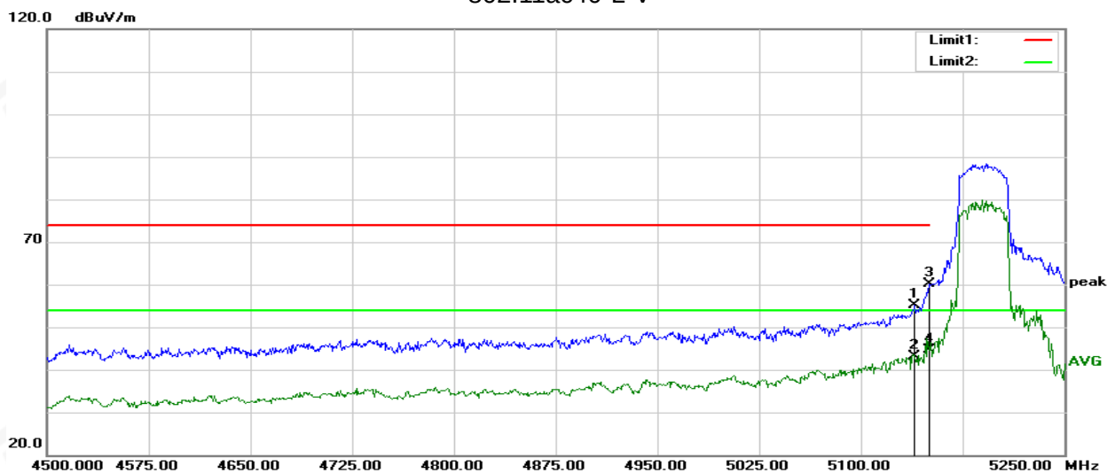
802.11ac40-L-V
