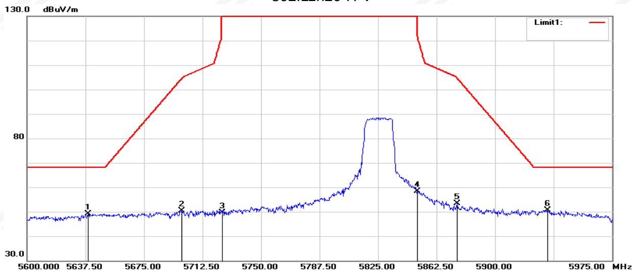
802.11n20-H-V
