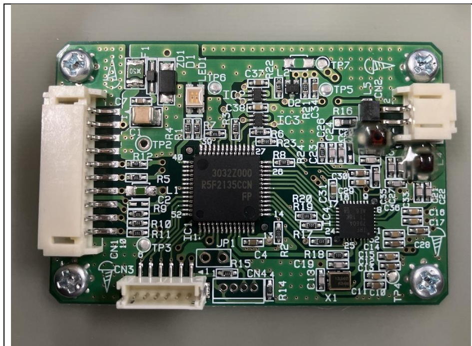
RFID reader module board_Front
