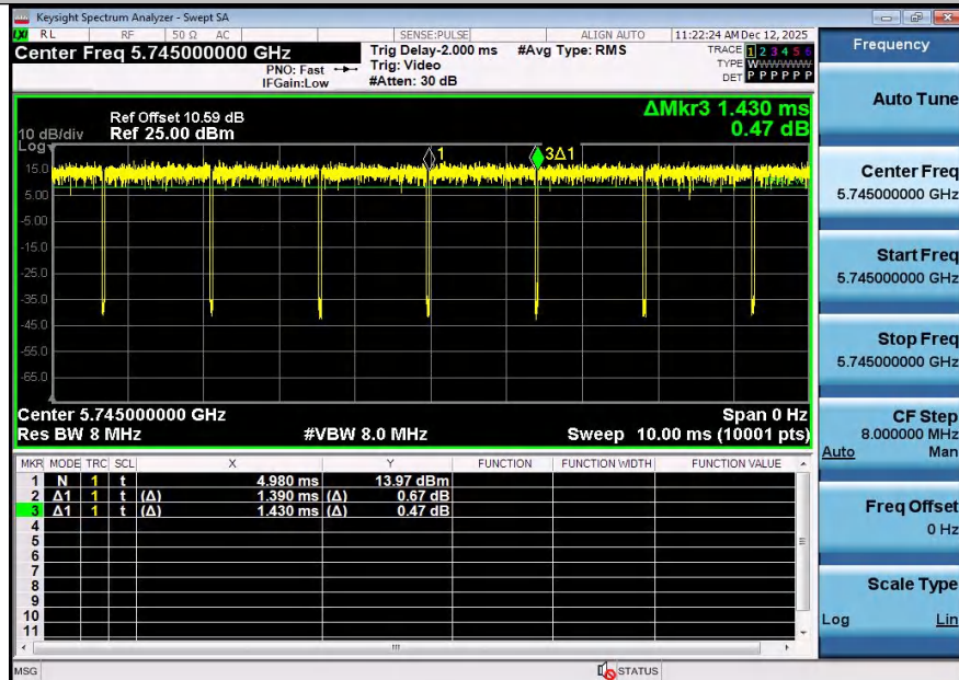
NTNV-11A-Ant1-5745
