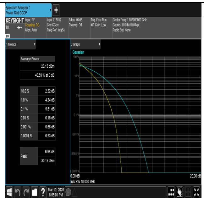
Band2-10MHz-QPSK-18650-50RB#0-PASS
