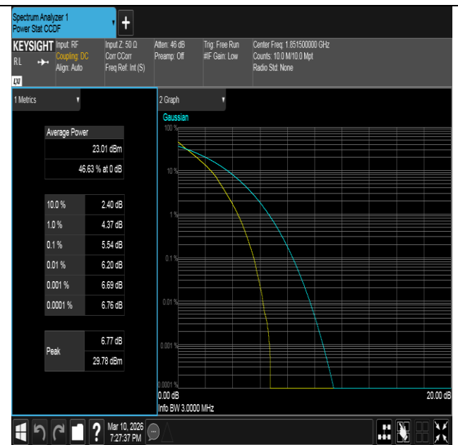
Band2-3MHz-QPSK-18615-15RB#0-PASS
