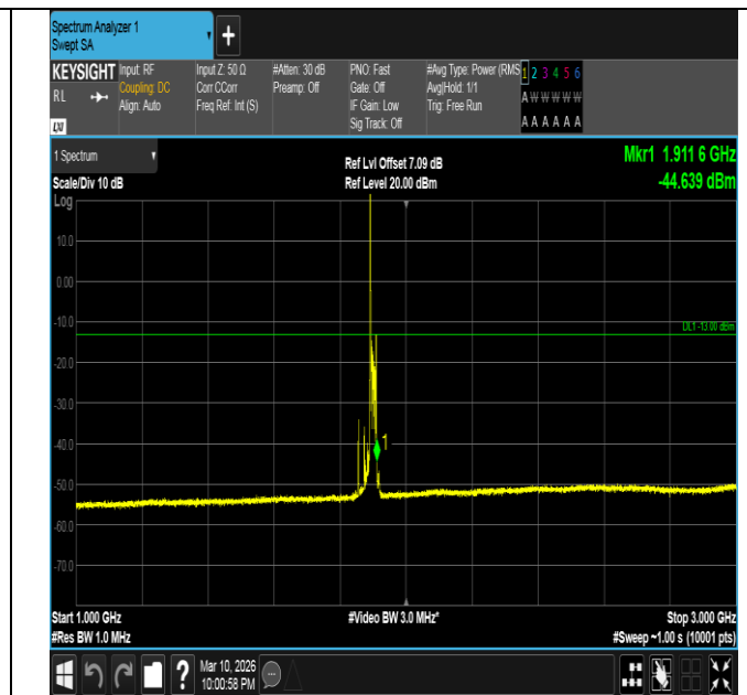
Band2-20MHz-QPSK-19100-1RB#0-1000~3000-PASS
