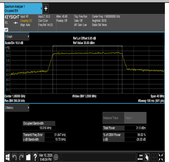
Band2-20MHz-16QAM-18700-100RB#0-PASS
