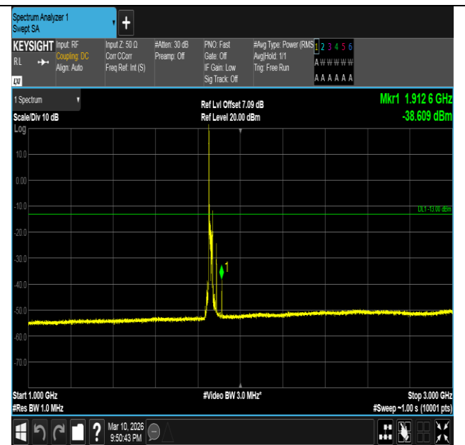
Band2-20MHz-QPSK-18700-1RB#0-1000~3000-PASS
