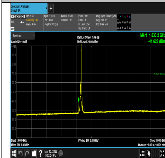
Band2-20MHz-QPSK-18700-1RB#99-1000~3000-PASS
