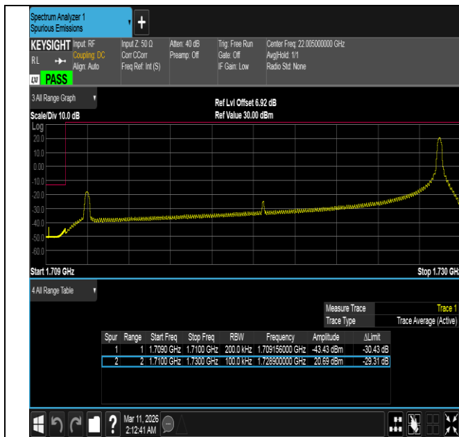
Band4-20MHz-16QAM-20050-1RB#99-PASS
