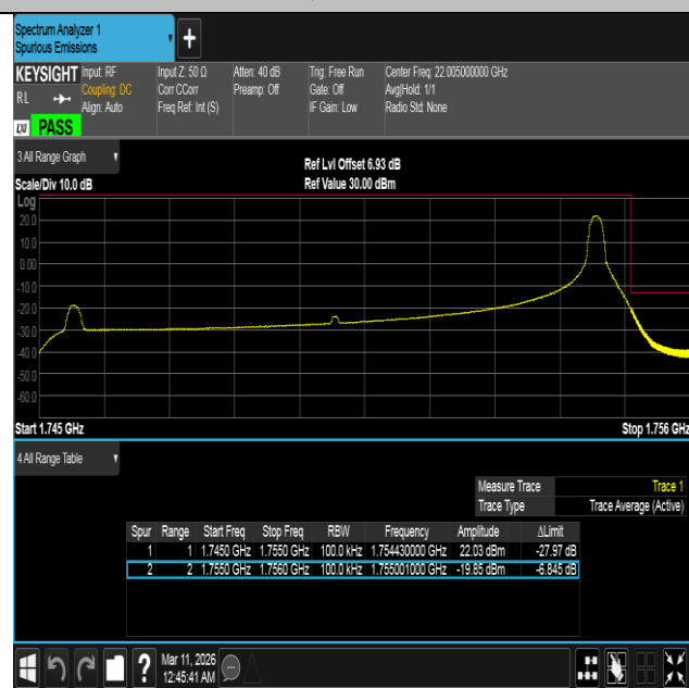
Band4-10MHz-QPSK-20350-1RB#49-PASS
