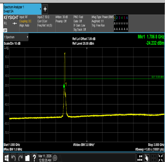
Band4-10MHz-QPSK-20000-50RB#0-1000~3000-PASS
