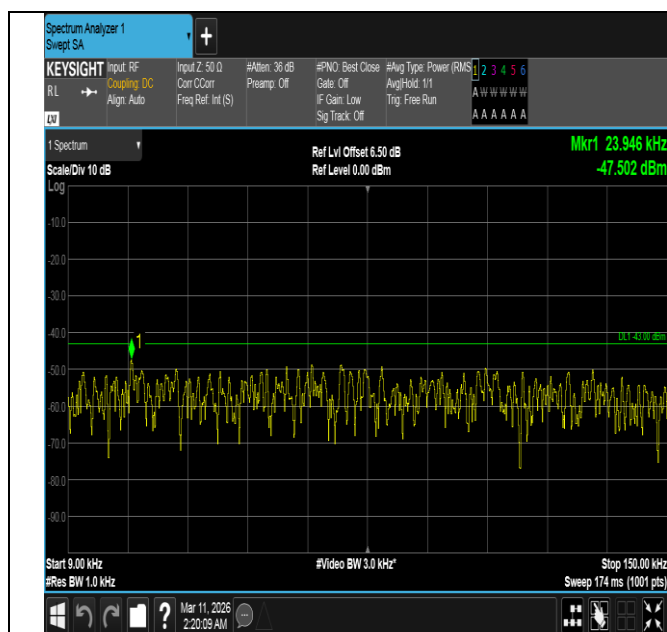
Band4-20MHz-QPSK-20175-1RB#0-0.009~0.15-PASS
