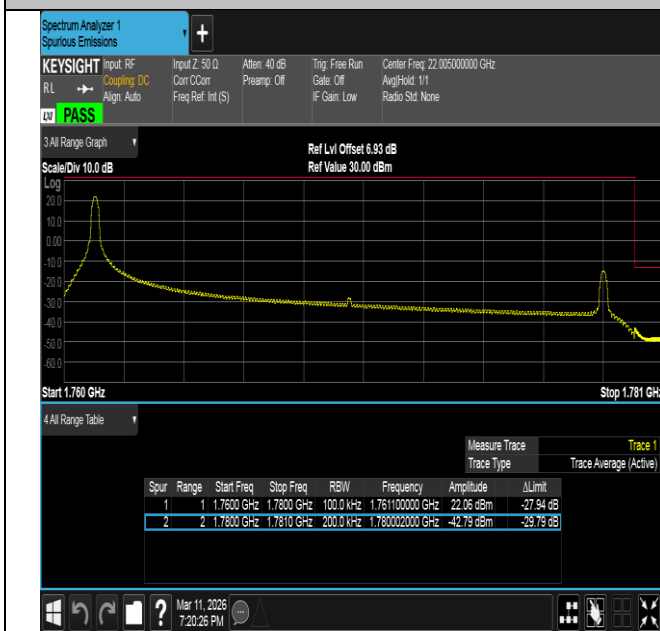
Band66-20MHz-QPSK-132572-1RB#0-PASS
