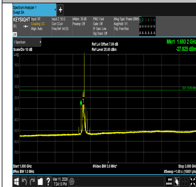
Band66-20MHz-QPSK-132072-1RB#99-1000~3000-PASS
