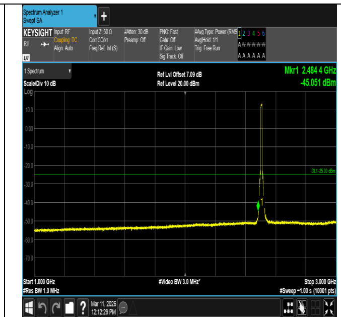
Band7-10MHz-QPSK-20800-50RB#0-1000~3000-PASS
