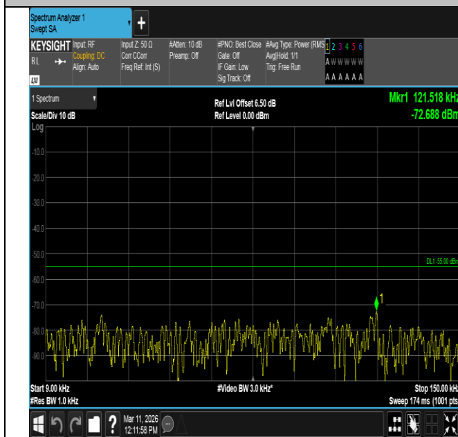
Band7-10MHz-QPSK-20800-50RB#0-0.009~0.15-PASS
