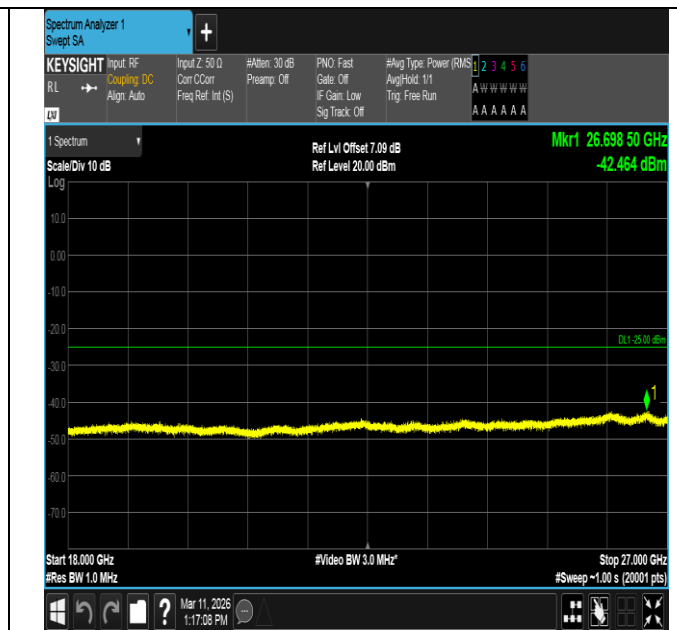
Band7-15MHz-16QAM-20825-1RB#0-18000~27000-PASS
