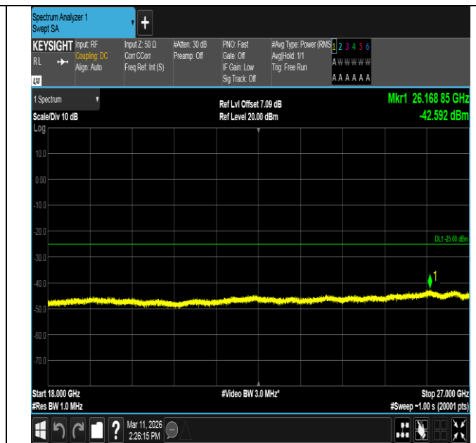
Band7-20MHz-QPSK-20850-1RB#99-18000~27000-PASS
