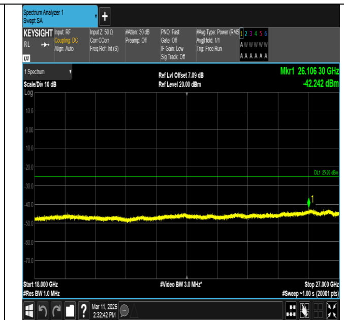
Band7-20MHz-QPSK-21100-1RB#99-18000~27000-PASS
