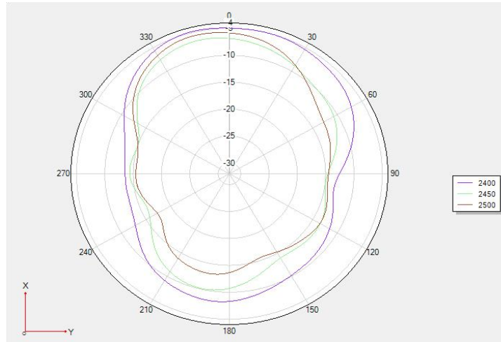
2400&2450&2500Mhz Theta=90 2D 图
