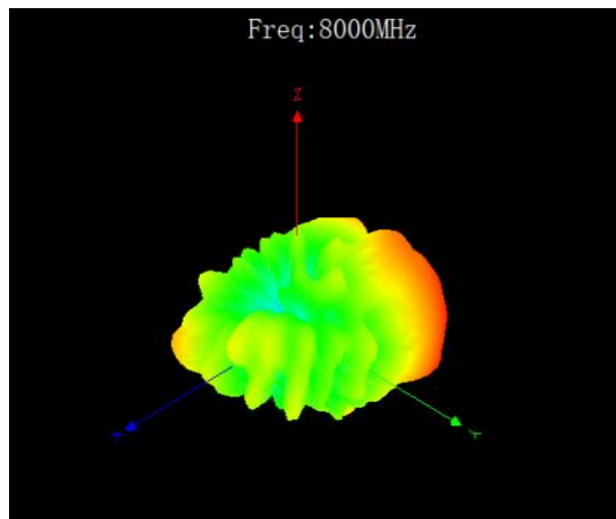
8000Mhz 3D 图
