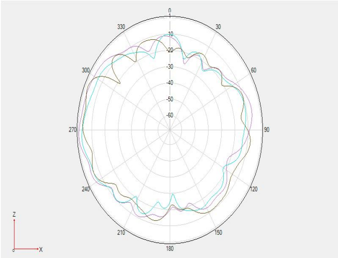
2400&2450&2500Mhz Phi=0 2D 图
