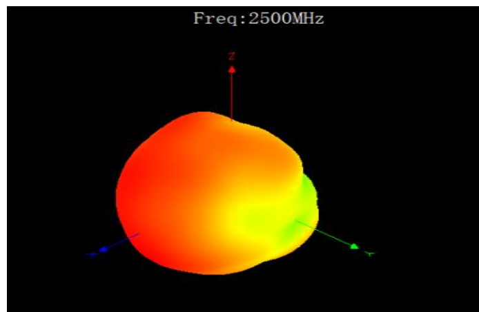
2500Mhz 3D 图
