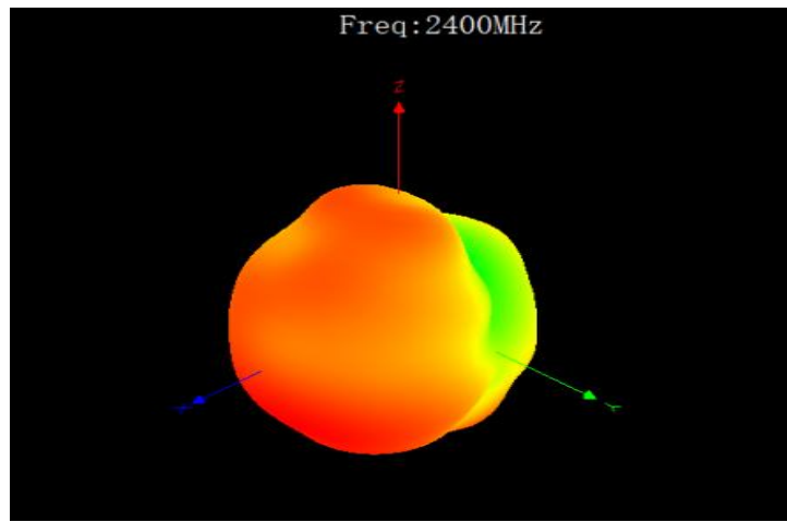
2400Mhz 3D 图
