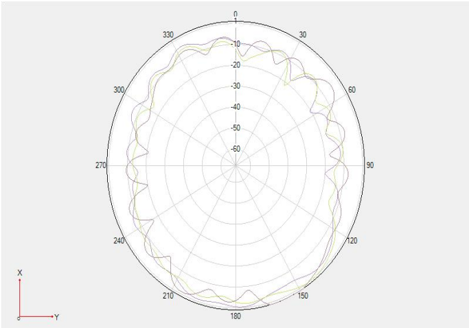
2400&2450&2500Mhz Theta=90 2D 图
