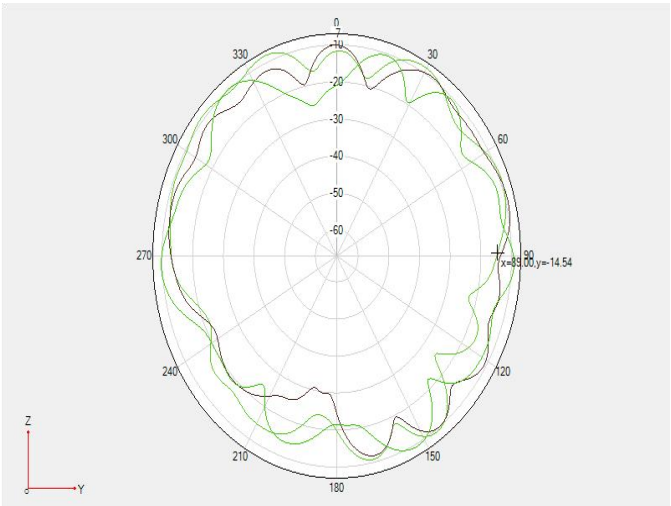
2400&2450&2500Mhz Phi=90 2D 图
