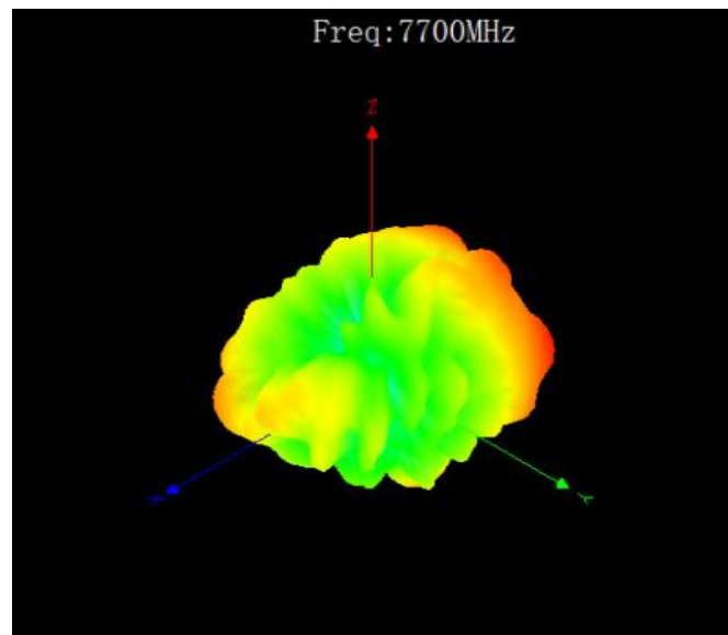
7700Mhz 3D 图
