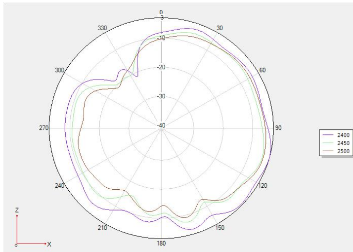
2400&2450&2500Mhz Phi=0 2D 图
