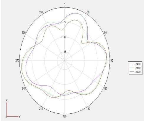
Theta=90
