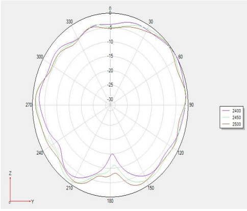
Phi=90
