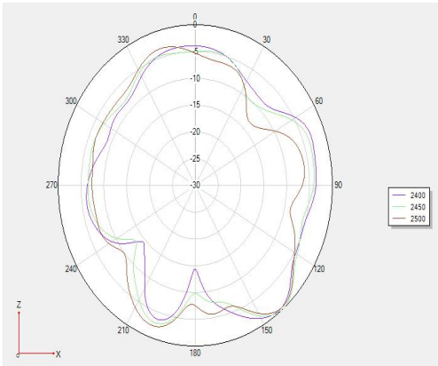
Phi=0
