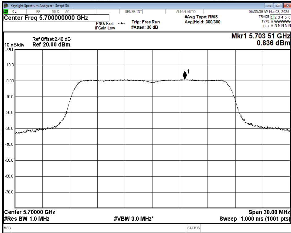
PSD NVNT a 5700MHz Ant1
