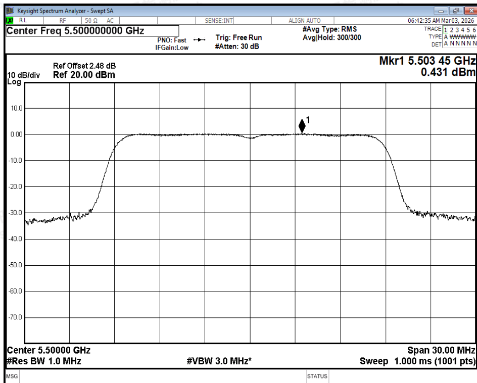
PSD NVNT n20 5500MHz Ant1
