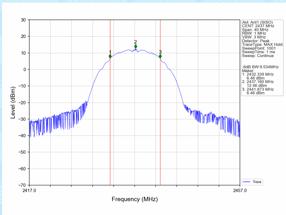
802.11b_MCH_2437MHz_Ant1 (SISO)_NTNV
