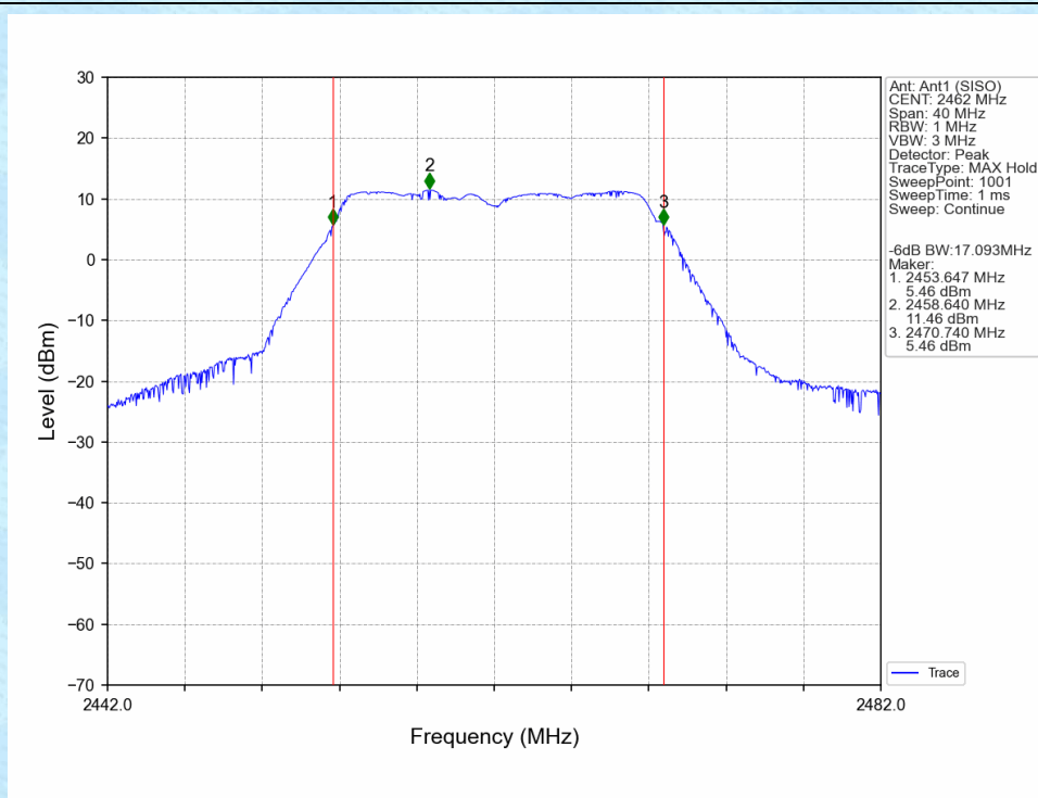
802.11g_HCH_2462MHz_Ant1 (SISO)_NTNV
