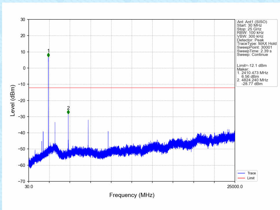
802.11b_LCH_2412MHz_Ant1 (SISO)_NTNV
