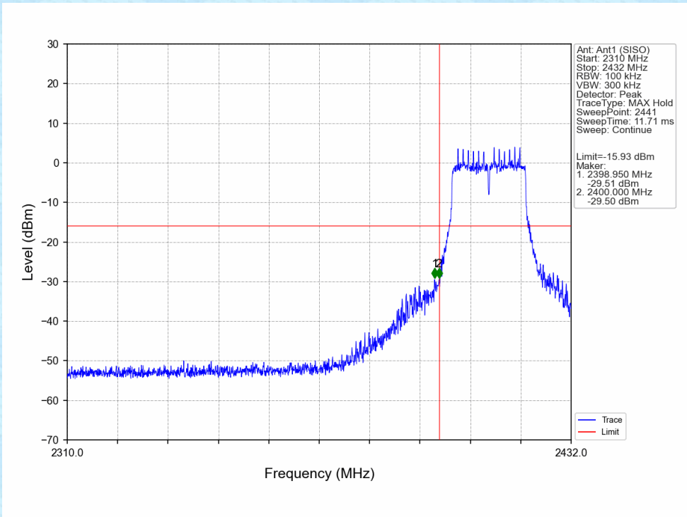
802.11n(HT20)_LCH_2412MHz_Ant1 (SISO)_NTNV
