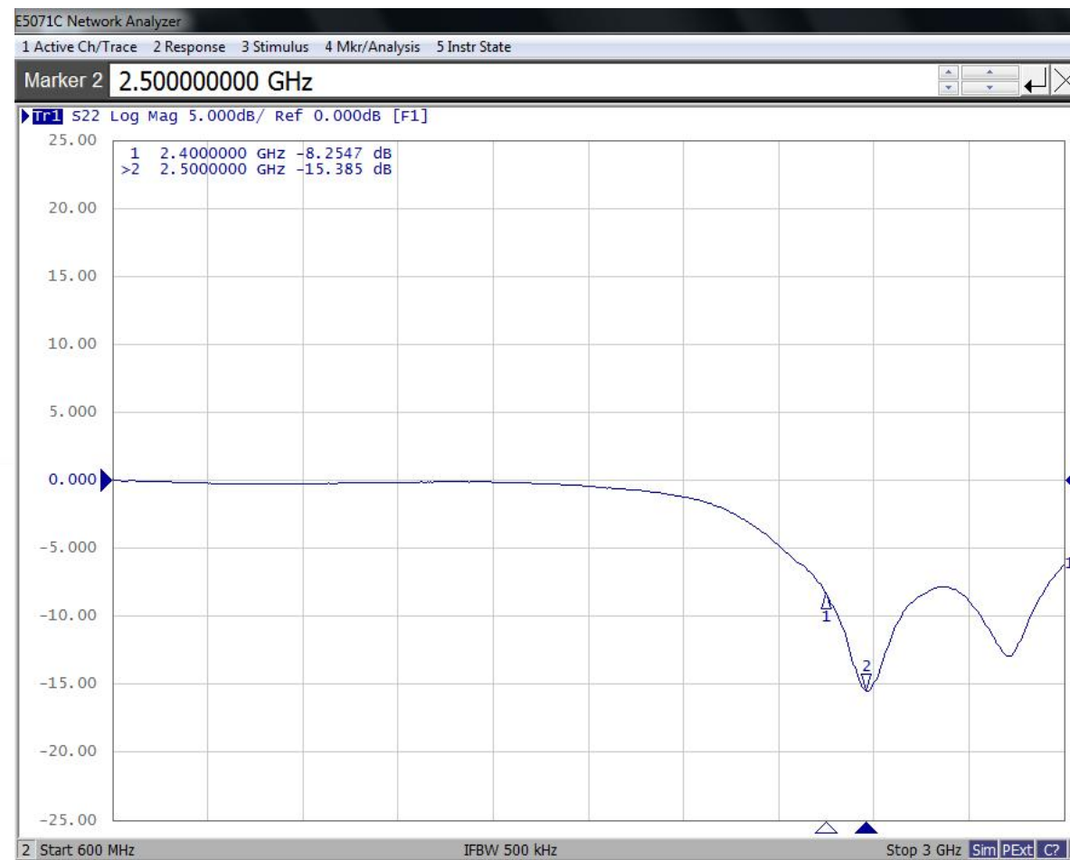
S-Parameter Test
