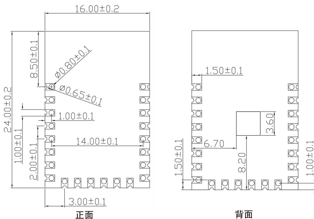
图 4 尺寸图
