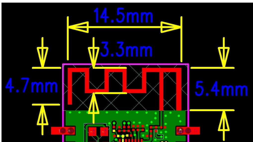
图 8 天线测试样机示意图
