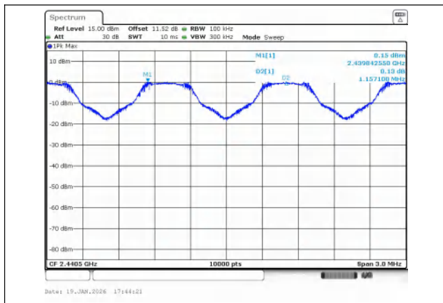
GFSK
