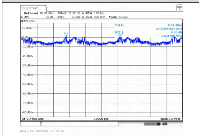
8DPSK
