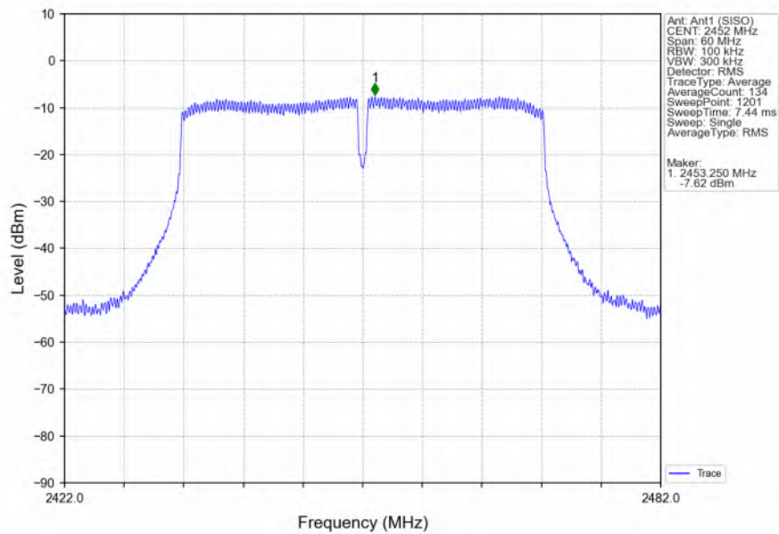
802.11n(HT40)_HCH_2452MHz_Ant1 (SISO)_NTNV
