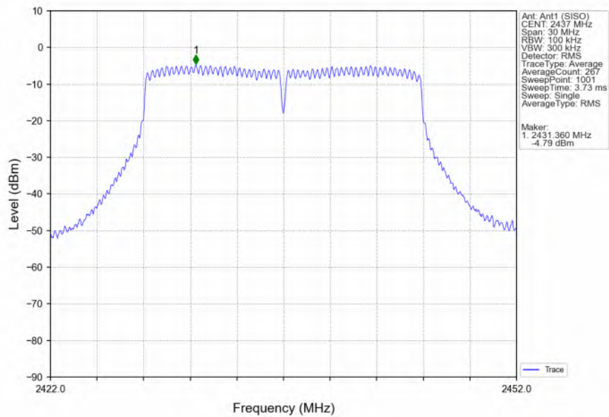
802.11n(HT20)_MCH_2437MHz_Ant1 (SISO)_NTNV
