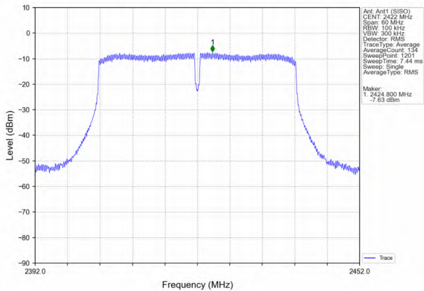
802.11n(HT40)_LCH_2422MHz_Ant1 (SISO)_NTNV
