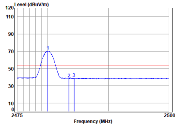
BLE_1M_TX_CH_39_Vertical-AVG
